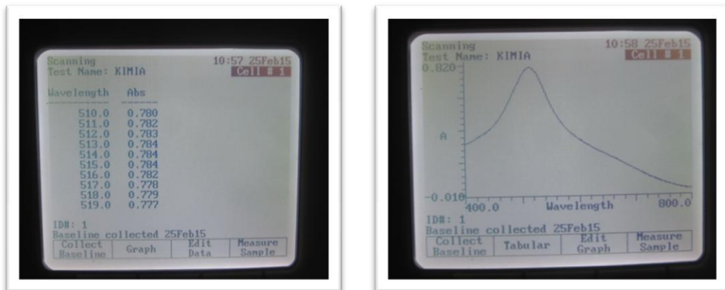
Gambar 6. Panjang gelombang maksimum DPPH
