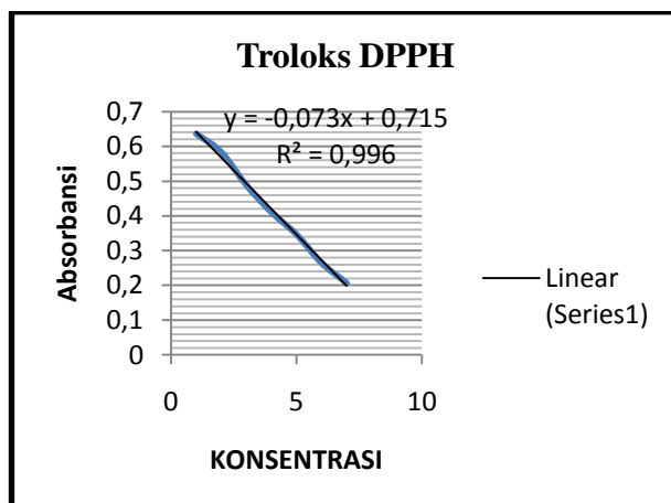
Gambar12. grafik absorbansi troloks metode DPPH
