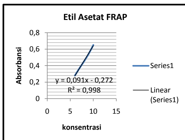
Gambar 18. grafik absorbansi ekstrak Etil Asetat metode FRAP
