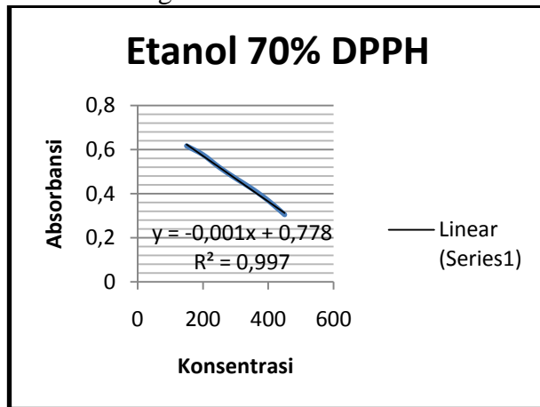
Gambar 11. grafik absorbansi Etanol 70% metode DPPH
