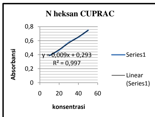
Gambar 13. grafik absorbansi n-heksan metode CUPRAC
