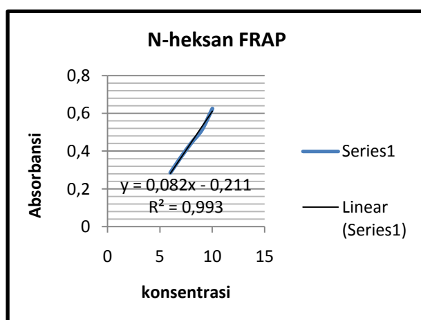
Gambar 17. grafik absorbansi ekstrak N-Heksan metode FRAP
