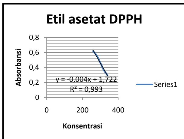
Gambar 10. grafik absorbansi etil asetat metode DPPH
