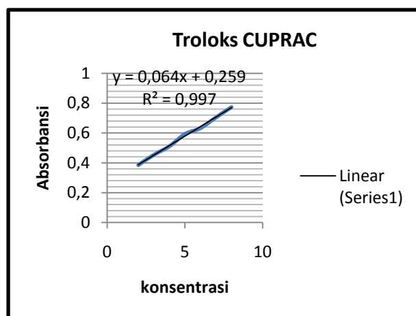
Gambar 16. grafik absorbansi troloks metode CUPRAC
