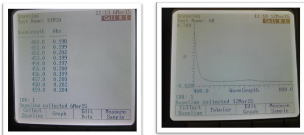
Gambar 7. Panjang gelombang maksimum CUPRAC
