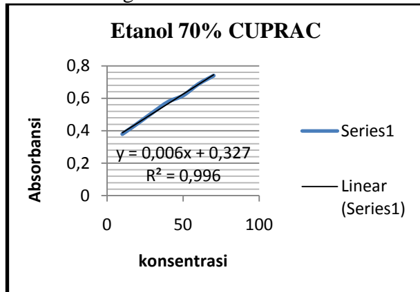
Gambar 15. grafik absorbansi Etanol 70% metodECUPRAC
