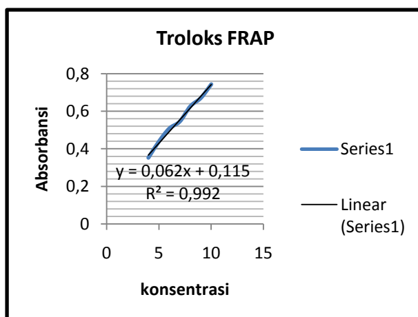
Gambar 20. grafik absorbansi Troloks metode FRAP
