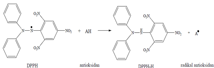
Gambar 2. Reaksi DPPH dengan Antioksidan (Molyneux, 2003)
