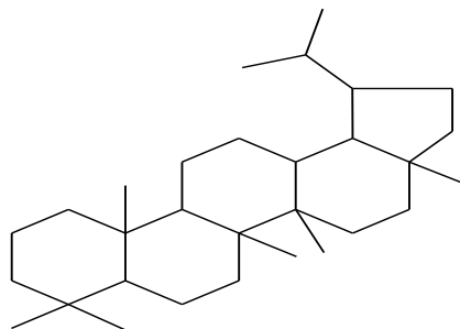
Gambar 2.3. Struktur Dasar Triterpen (Ilyas, 2013: 37-38).
