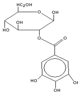
Gambar 2.6. Struktur Tannin Acid (Sumber: Ismarani, 2012: 51).
