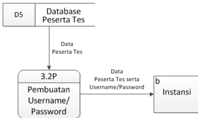
Gambar 4. 25. DFD Level 2 Proses 3.2
