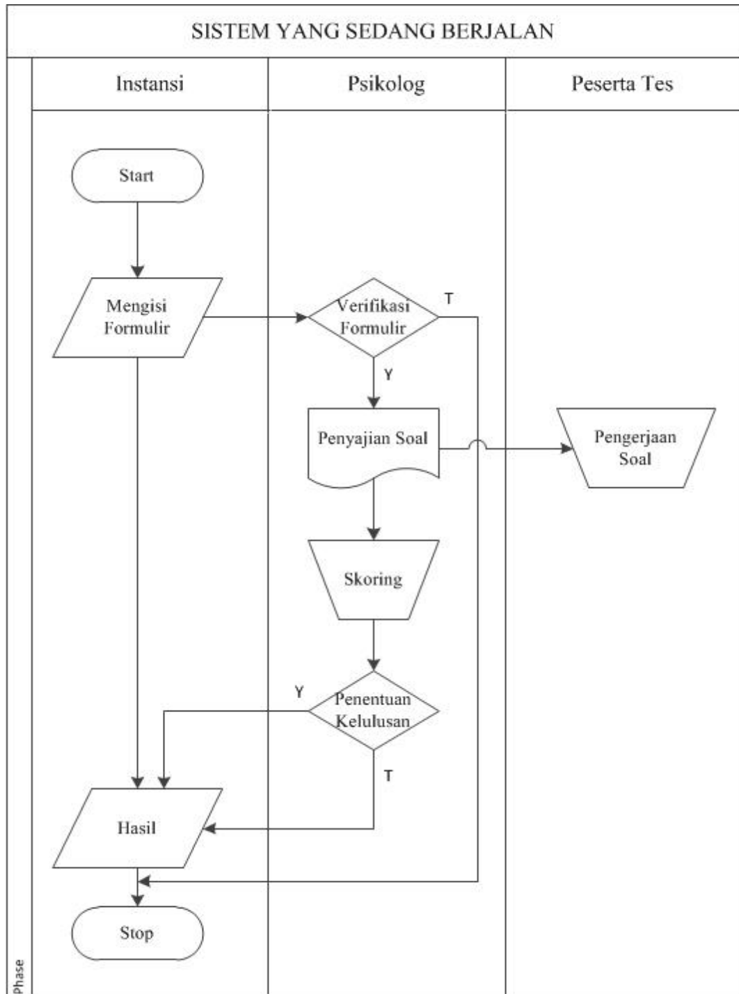
Gambar 4. 1. Bagan Alir Sistem yang Sedang Berjalan
