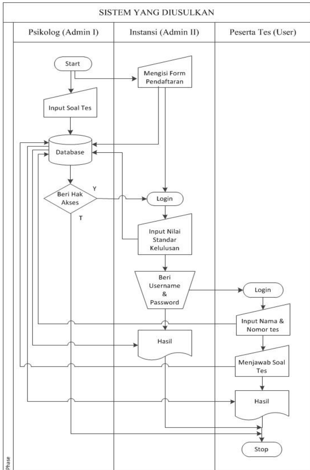
Gambar 4. 2. Bagan Alir Sistem yang Diusulkan
