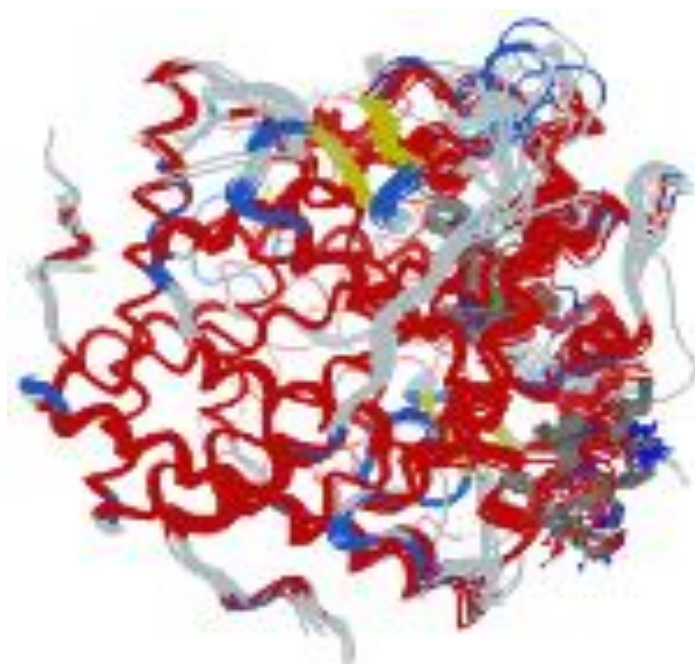
Gambar IV. 5 Struktur protein sejajar di style ribbon dalam bentuk line
