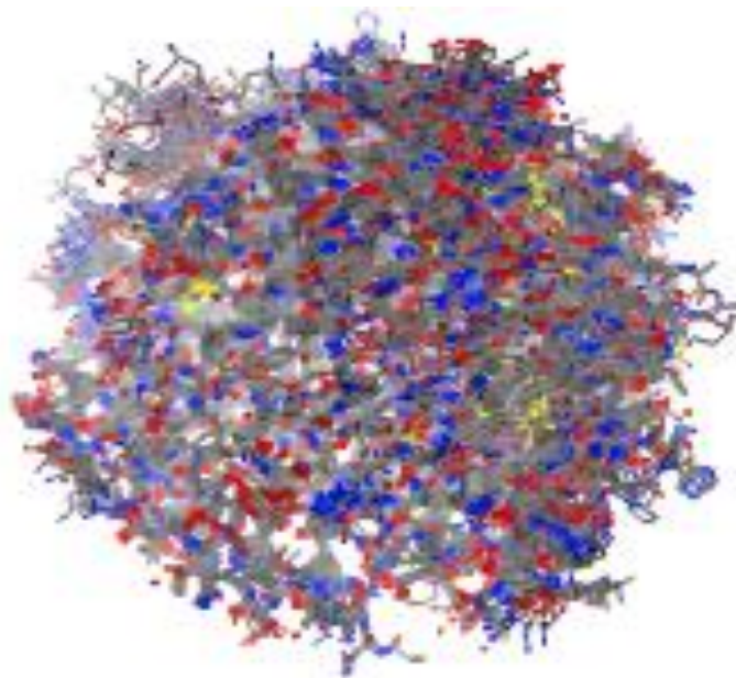
Gambar IV. 3 Struktur Protein setelah disejajarkan ( Superpose )
