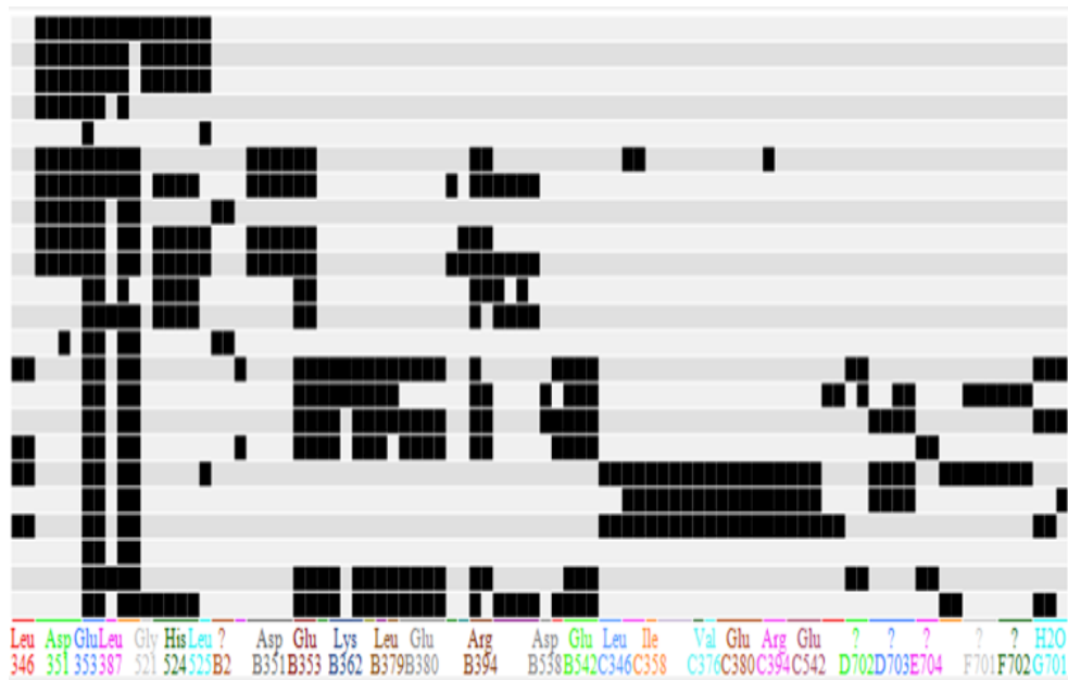
Gambar IV.1 Interaksi Ligan dengan Asam Amino
