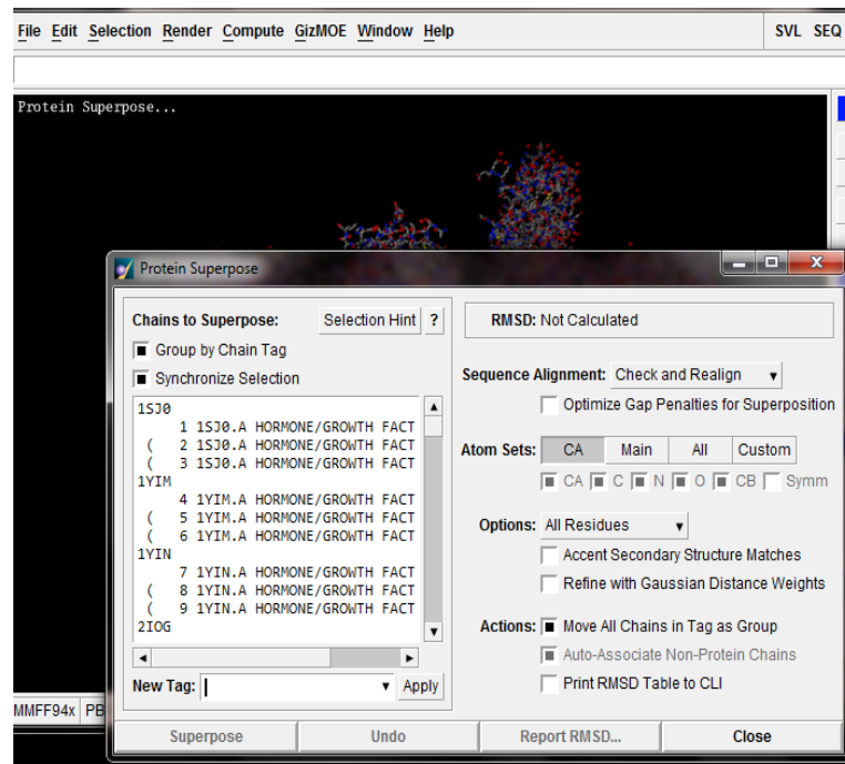
Gambar IV.2 Struktur Protein di Superpose
