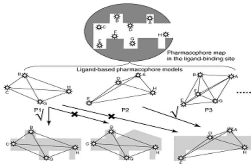
Gambar II.4 Pendekatan berbasis struktur dan model farmakofor
