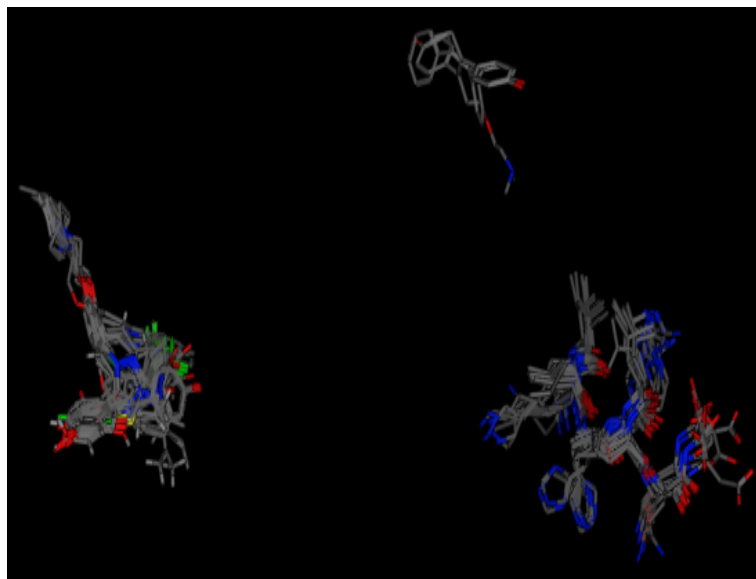
Gambar IV. 4 Struktur Protein setelah di Show Ligan
