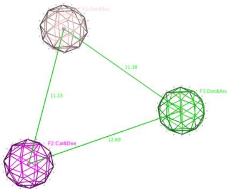
Gambar IV.7 Jarak antar fitur-fitur dalam farmakofor query
