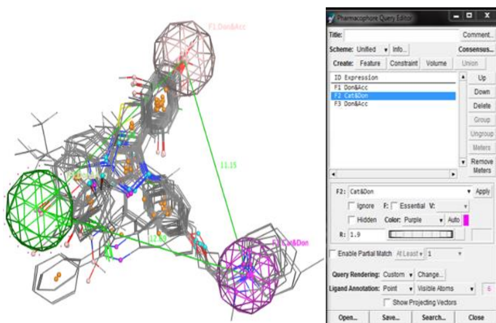
Gambar IV.6 Fitur Farmakofor dan Query Editor
