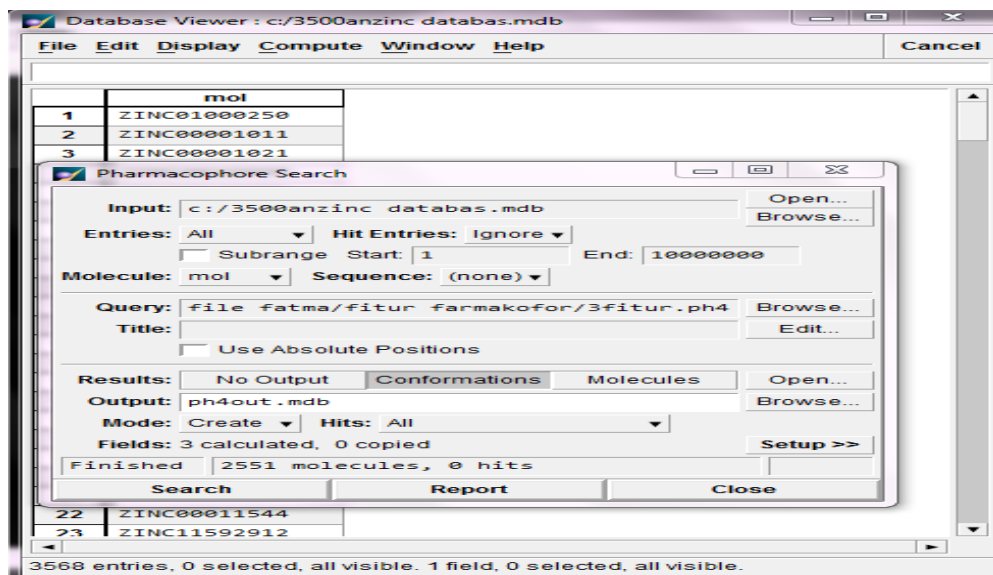
Gambar III.7 Tampilan skrining zinc databes dengan fitur farmakofor
