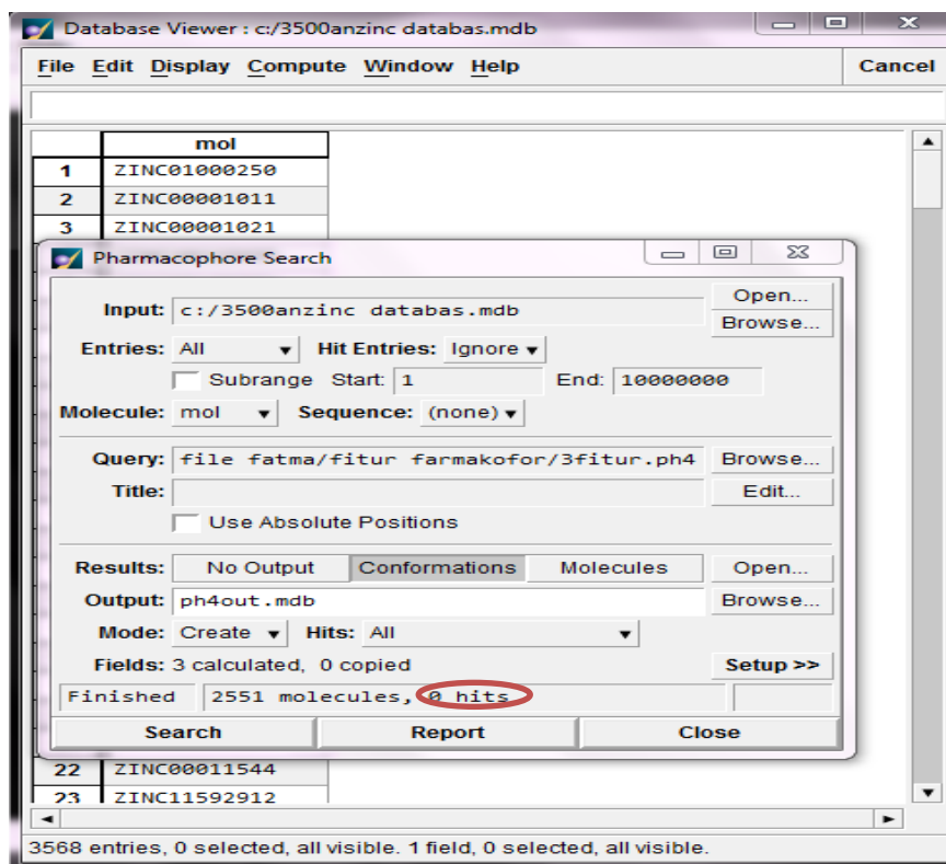
Gambar IV.8 Virtual Skrining Fitur Farmakofor dengan 3568 Senyawa
