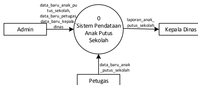
Gambar IV. 3 Diagram Konteks Sistem Pendataan Anak Putus Sekolah
