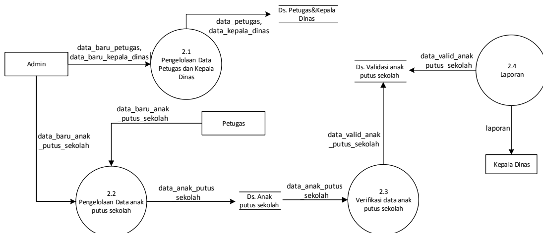
Gambar IV. 5 DFD level 1 Sistem Pendataan Anak Putus Sekolah
