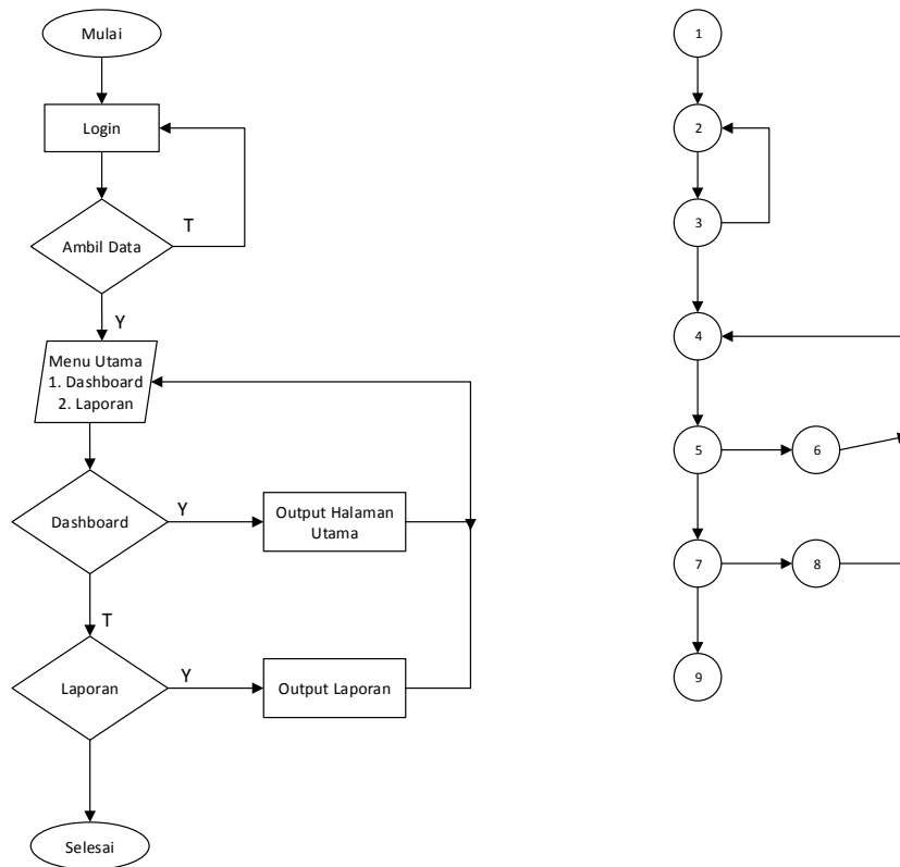
Gambar V. 20 Pengujian white box sebagai Kepala Dinas
