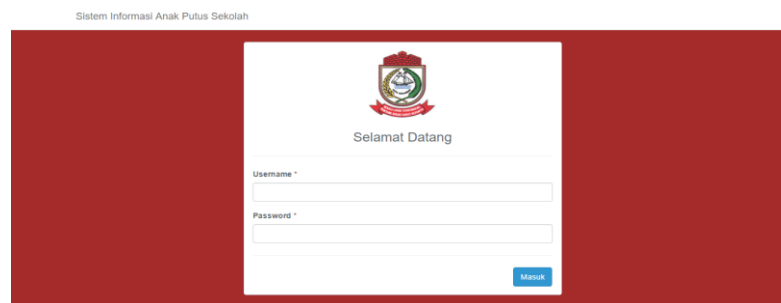
Gambar V. 17 Antarmuka Login
