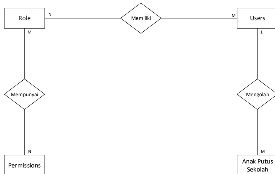
Gambar IV. 6 ERD Sistem Pendataan Anak Putus Sekolah
