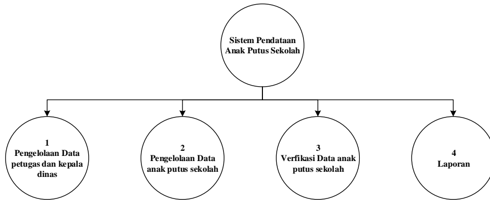
Gambar IV. 4 Diagram Berjenjang Proses Sistem Pendataan Anak Putus Sekolah
