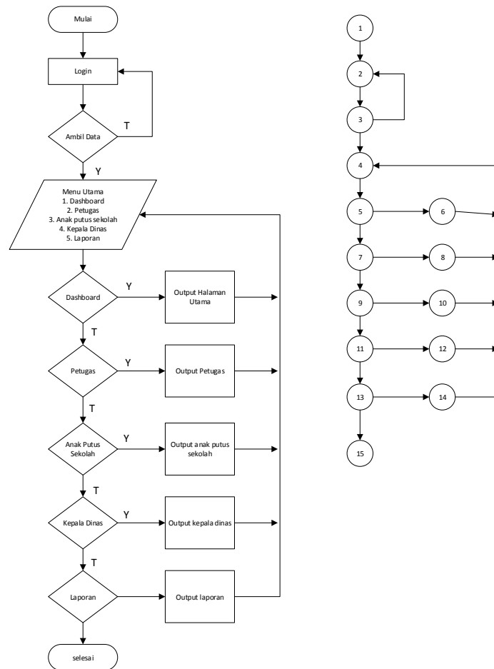
Gambar V. 18 Pengujian white box sebagai admin
