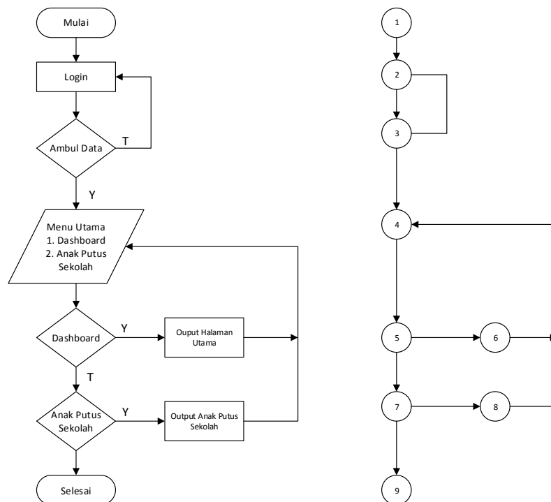
Gambar V. 19 Pengujian white box sebagai petugas
