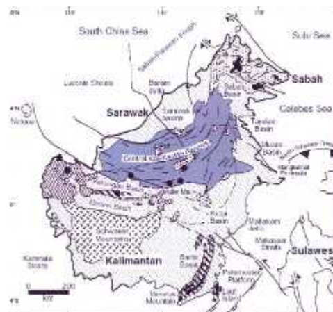
Gambar 5. Peta geologi pulau Kalimantan
