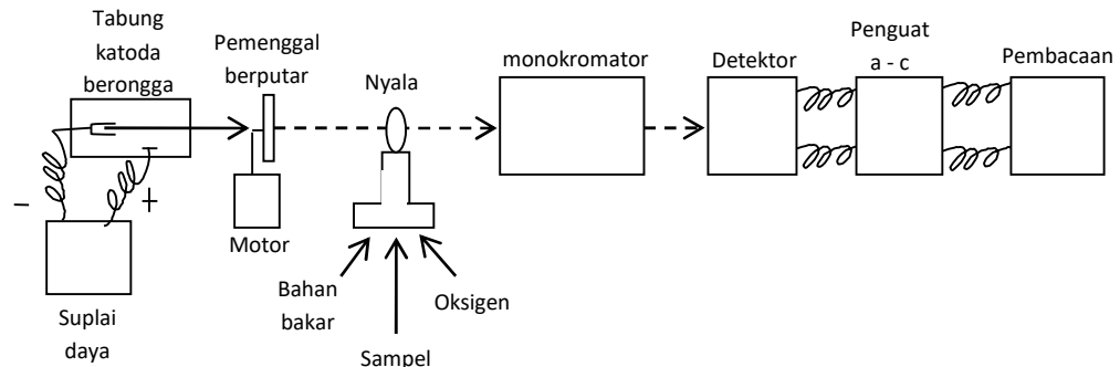
Gambar 3. Komponen-komponen suatu spektrofotometer serapan atom (Day & Underwood, 2002:425).
