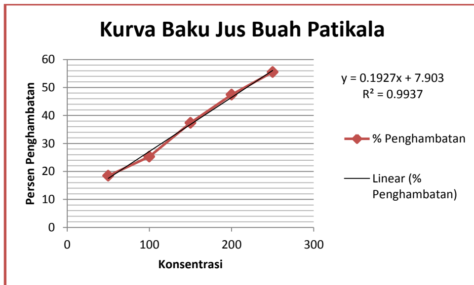
Gambar 12. Jus Buah Patikala terhadap DPPH
