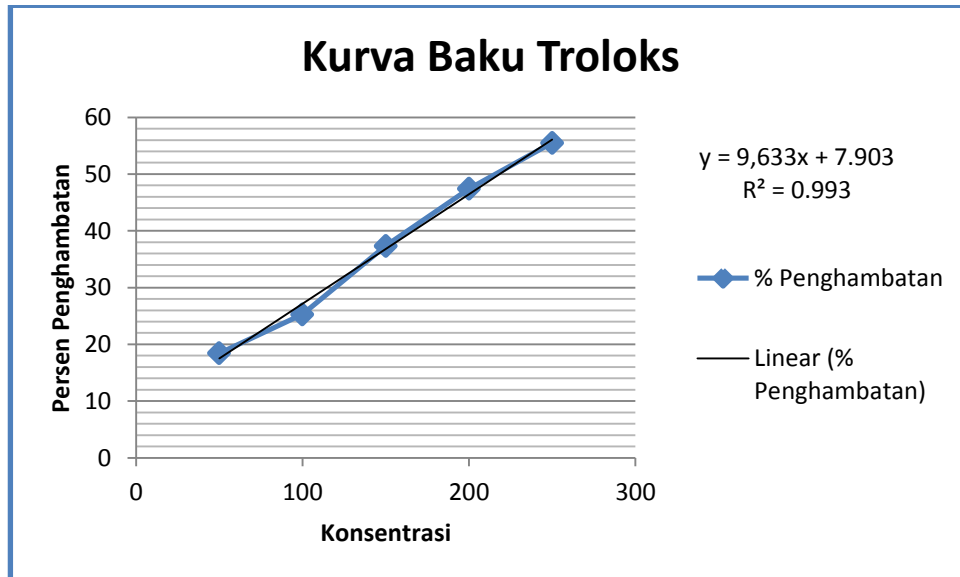
Gambar 11. Troloks terhadap DPPH
