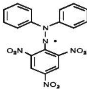
Gambar 2. Rumus Bangun DPPH
