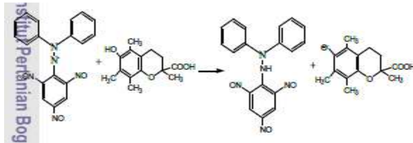
Gambar 6. Reaksi penangkapan atom H oleh DPPH dari Troloks ®
