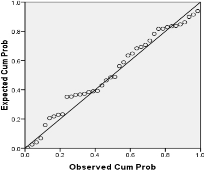
Grafik Normal P-Plot
