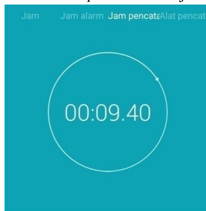
Gambar 4.5 : Stopwatch Peminjaman
