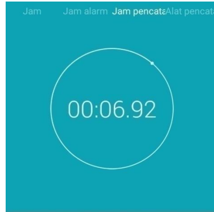
Gambar 4.7 Stopwatch Peminjaman
