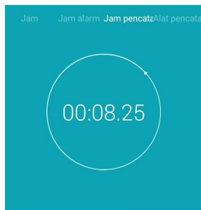
Gambar 4.6 Stopwatch Peminjaman
