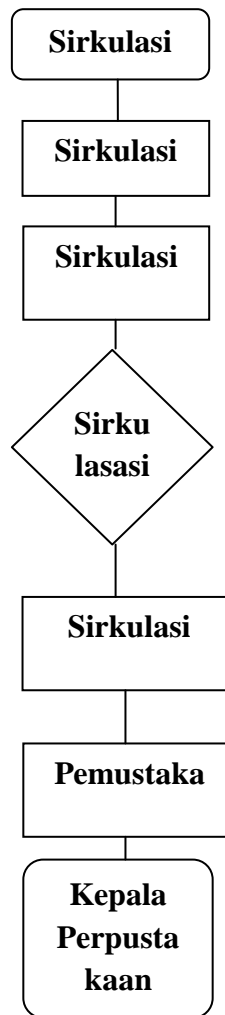
Gambar 4.3 Flowchat Peminjaman
