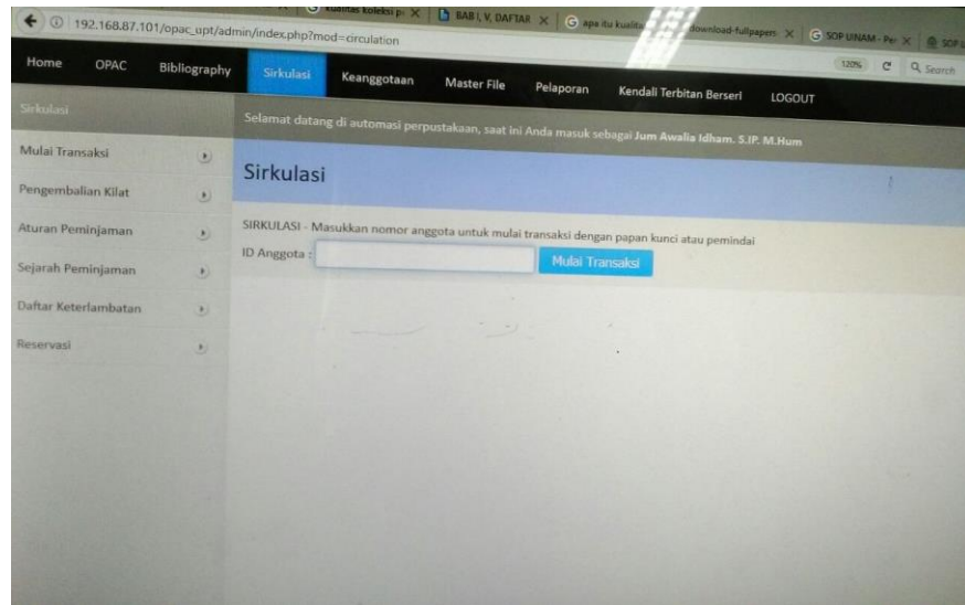
Gambar 4.1 Modul sirkulasi
