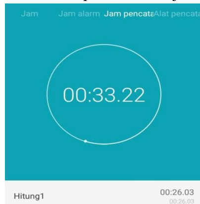
Gambar 4.4 Stopwatch Peminjaman
