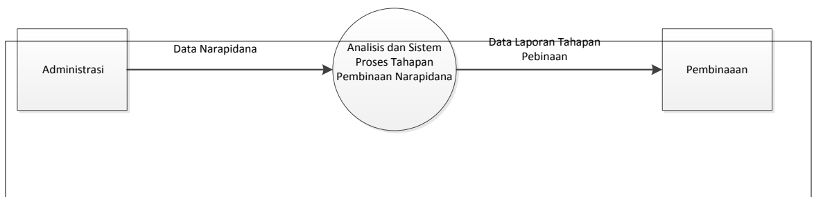
Gambar. IV.1 Diagram Konteks
