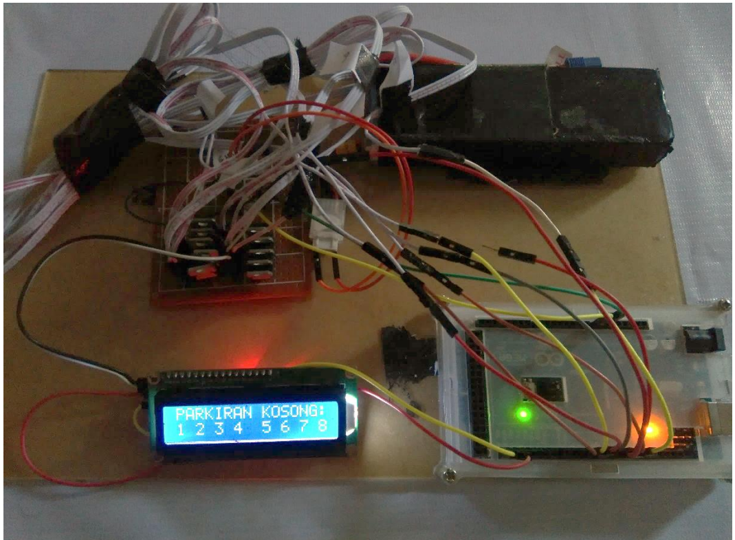
Gambar V.2 Rancangan Sistem Alat Sistem Informasi parkir
