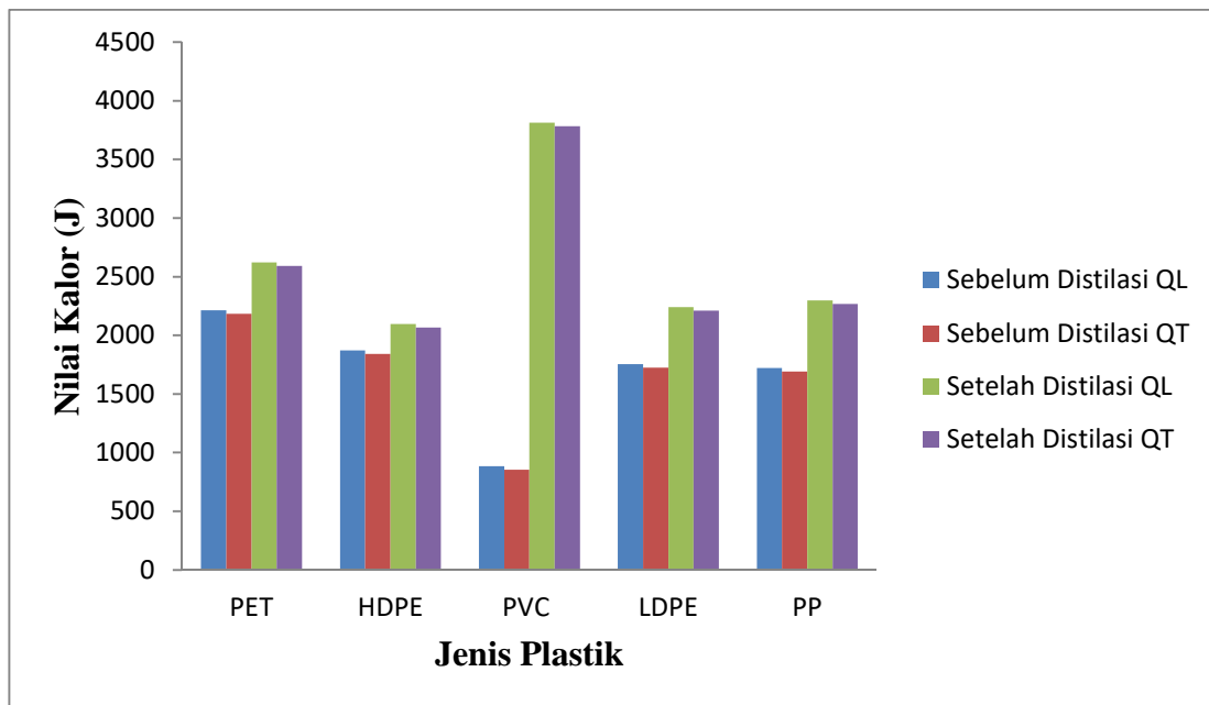
Grafik IV.3 Pengujian Nilai Kalor Beberapa Jenis Plastik
