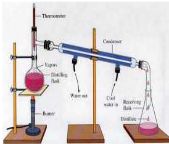
Gambar II.8 Rangkaian Alat Distilasi Sederhana
