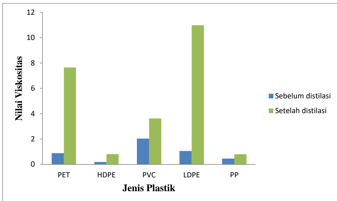
Grafik IV.2 Pengujian Viskositas Beberapa Jenis Plastik
