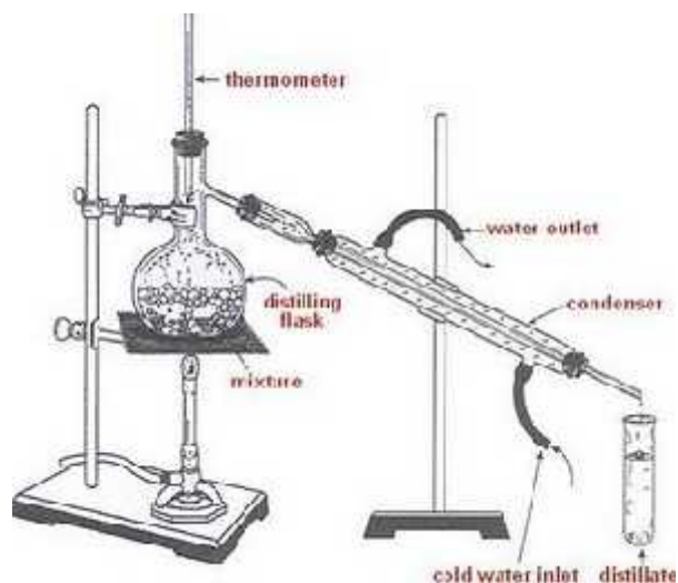
Gambar II.9 Rangkaian Alat Distilasi Fraksionisasi
