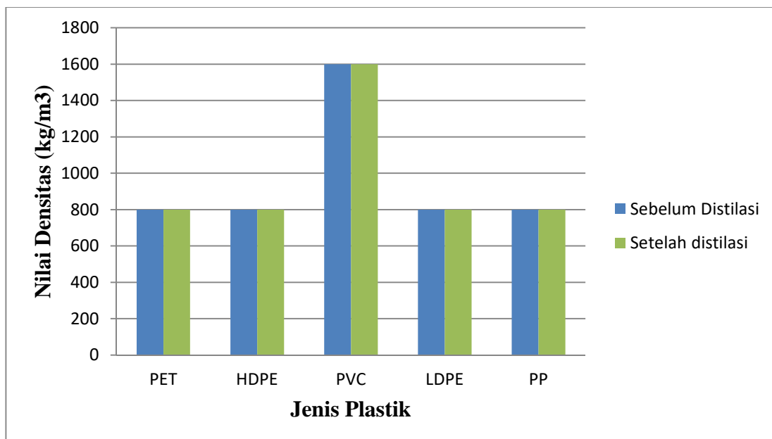
Grafik IV.1 Pengujian Densitas Beberapa Jenis Plastik
