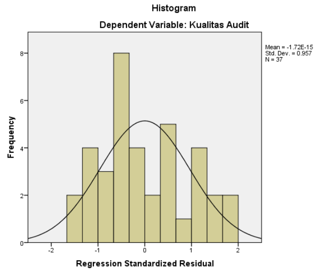
Gambar 4.1 Grafik Histogram
