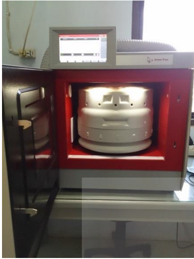
Gambar 12 Persiapan destruksi
