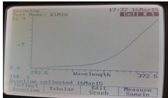
Gambar 25. Grafik transmisi formulasi III (Replikasi 2)
