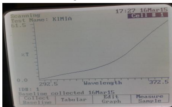
Gambar 23. Grafik transmisi formulasi II (Replikasi 3)
