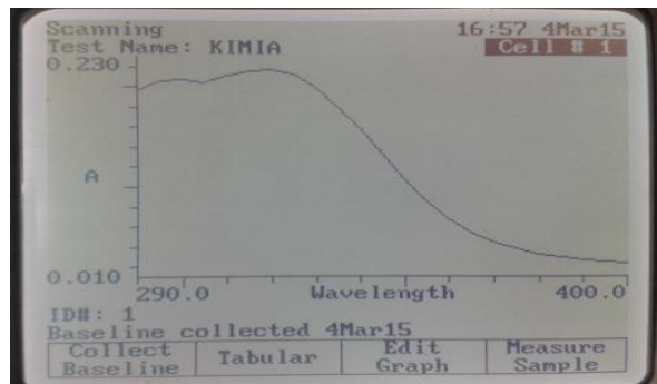
Gambar 10. Grafik absorbansi ekstrak konsentrasi 0,02 %
