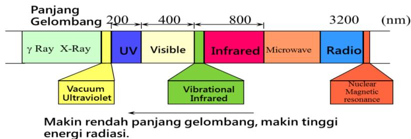
Gambar 2. Spektrum Elektromagnetik (Bismo, 2006: 6)
