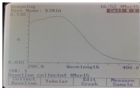
Gambar 9. Grafik absorbansi ekstrak konsentrasi 0,01 %
