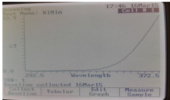
Gambar 27. Grafik transmisi formulasi IV (Replikasi 1)
