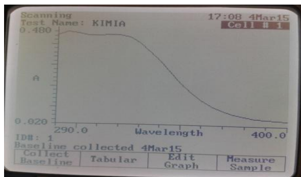
Gambar 12. Grafik absorbansi ekstrak konsentrasi 0,04 %
