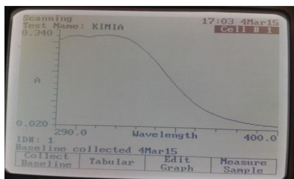
Gambar 11. Grafik absorbansi ekstrak konsentrasi 0,03 %
