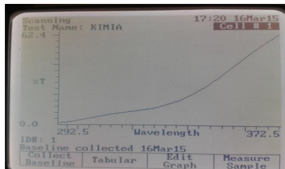
Gambar 22. Grafik transmisi formulasi II (Replikasi 2)
