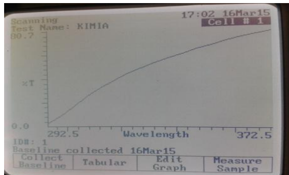
Gambar 19. Grafik transmisi formulasi I (Replikasi 1)
