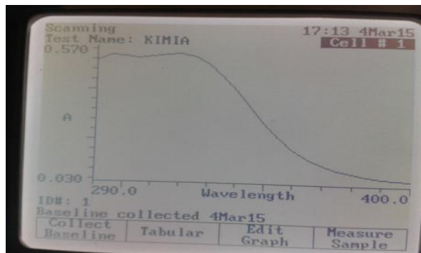
Gambar 13. Grafik absorbansi ekstrak konsentrasi 0,05 %
