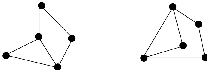
Gambar 2.19 Graf G_1 dan G_2
