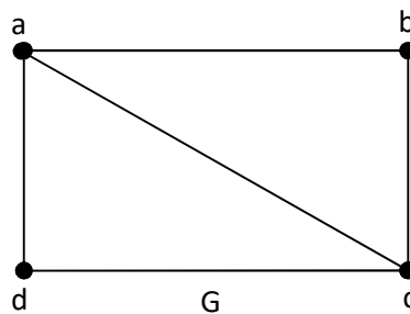
Gambar 2.4 Derajat
