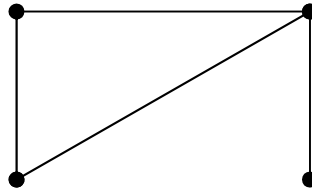
Gambar 2.7 Sirkuit v_1-v_2-v_3-v_1
