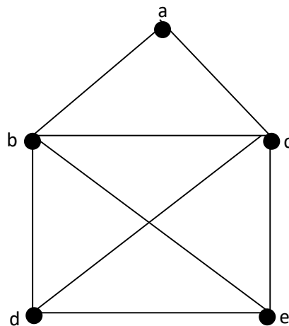
Gambar 2.20 Graf
