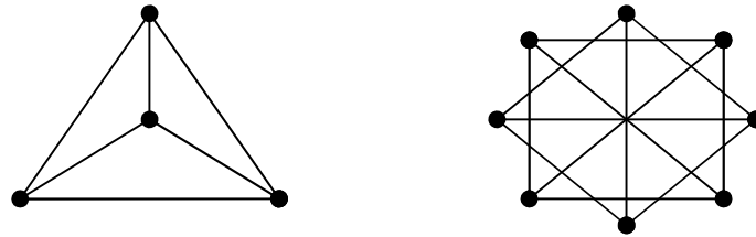
Gambar 2.12 Graf kubik
