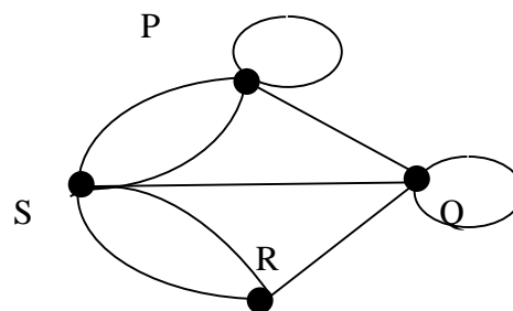
Gambar 2.5 graf
