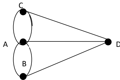
Gambar 1.2 Ilustrasi jembatan Konigsberg
