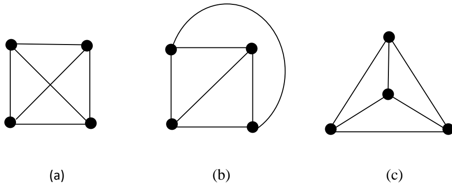
Gambar 2.22 Tiga buah graf planar, graf (b) dan (c) adalah graf bidang
