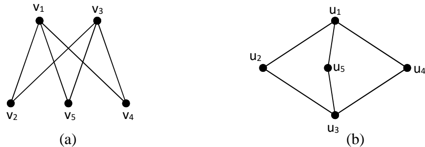
Gambar 2.16 graf
