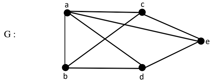
Gambar 2.14 graf G
