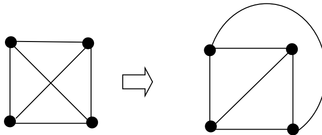
Gambar 2.20 K_4 adalah graf planar
