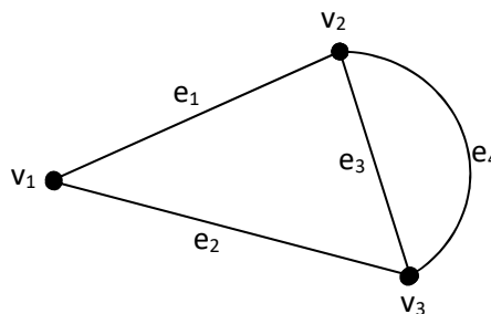
Gambar 2.1 Graf H_1
