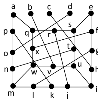
Gambar 4.7 Graf Nauru ( G_3 )
