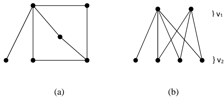
Gambar 2.10 (a) graf bipartit dan (b) partisi graf bipartit
