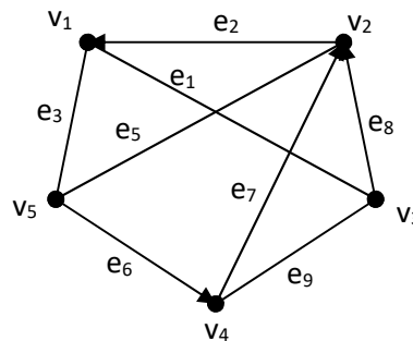
Gambar 2.6 lintasan
