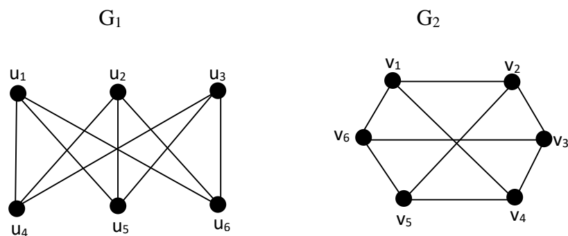
Gambar 2.18 graf isomorfik
