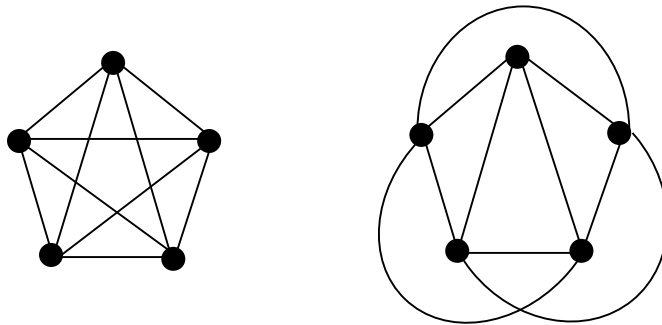
Gambar 2.21 K_5 bukan graf planar
