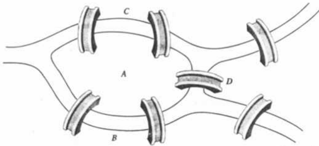
Gambar 1.1. Masalah Jembatan Königsberg
