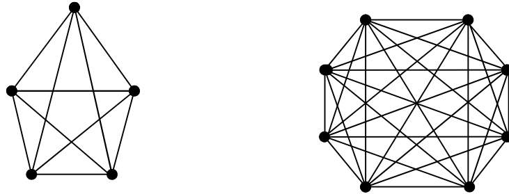
Gambar 2.9 graf lengkap
