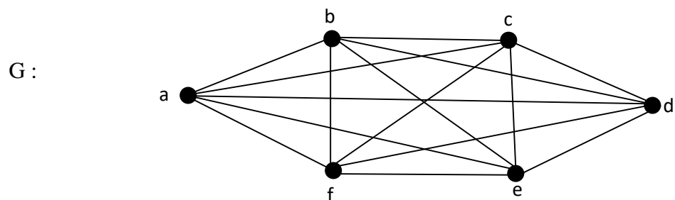
Gambar : 2.15 graf G
