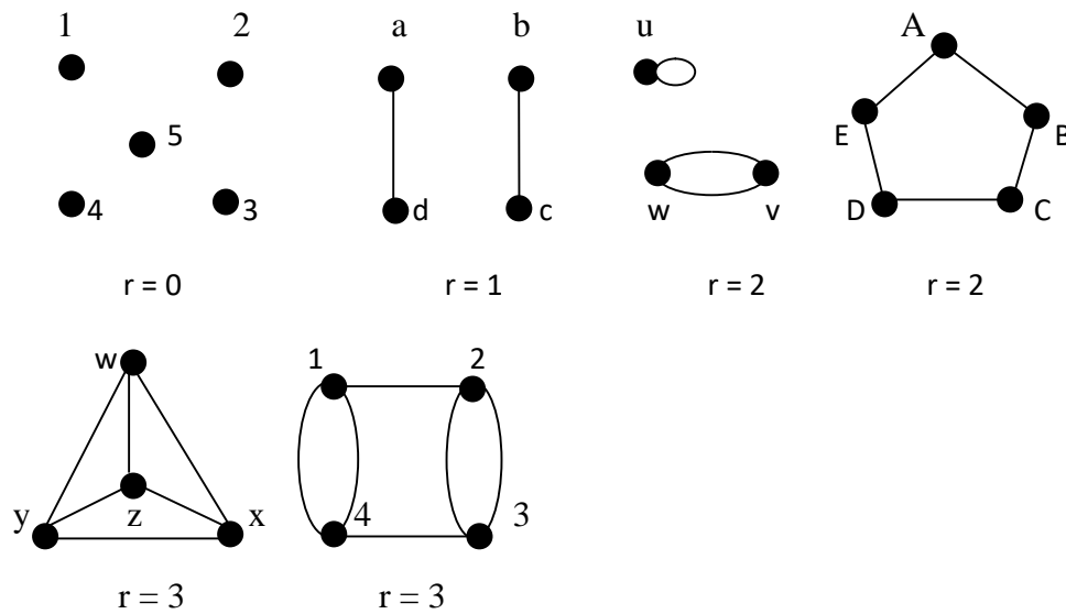
Gambar 2.8 graf teratur
