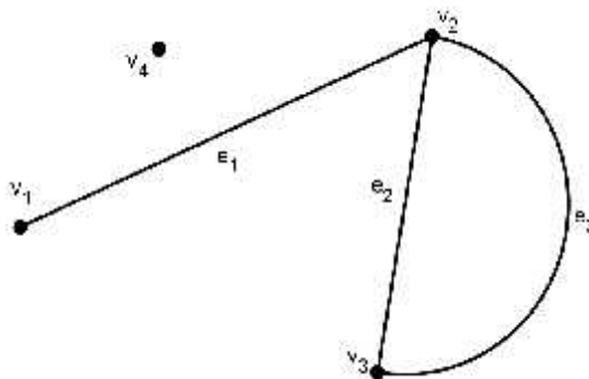
Gambar 2.3 multigraf G_2
