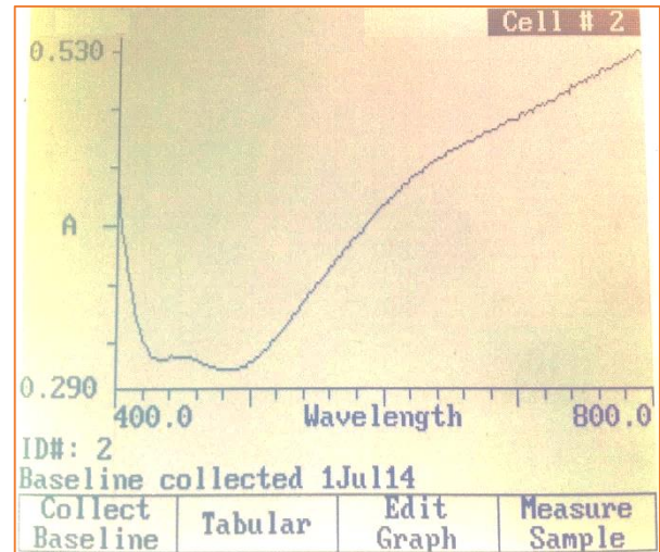
Gambar 13. Kurva absorbansi panjang gelombang maksimum Larutan asam galat
