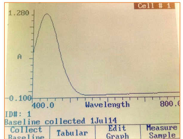
Gambar 14 kurva abserbansi panjang gelombang maksimum larutan kursetin
