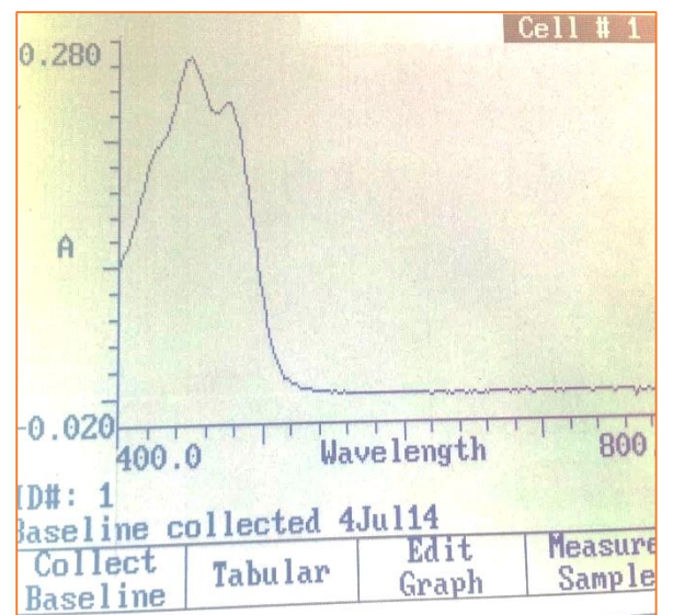
Gambar 16. Kurva absorbansi panjang gelombang maksimum beta karotenoid
