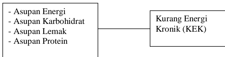
Gambar 2. Kerangka Konsep
