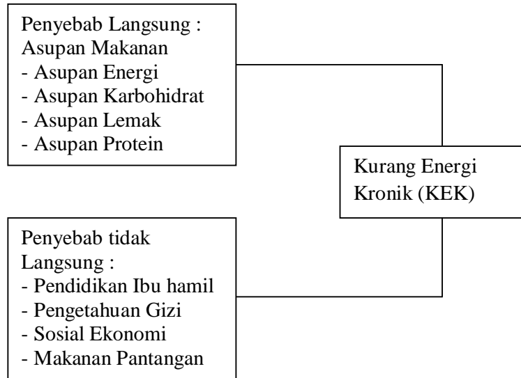
Gambar 1. Kerangka Teori
