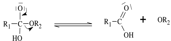
Gambar 3. Saponifikasi tahap II
