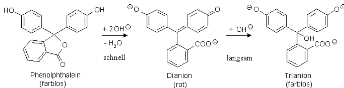
Gambar 7. Reaksi phenophthalein dengan NaOH
