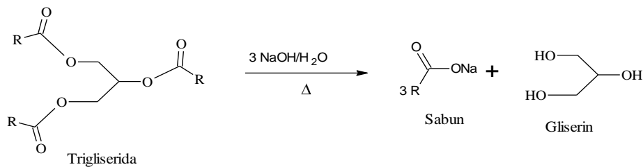
Gambar 5. Proses terbentuknya sabun (penyabunan) atau saponifikasi.
