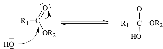
Gambar 2. Saponifikasi tahap I
