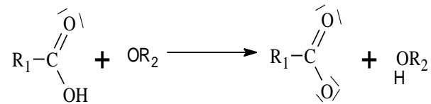
Gambar 4. Saponifikasi tahap III
