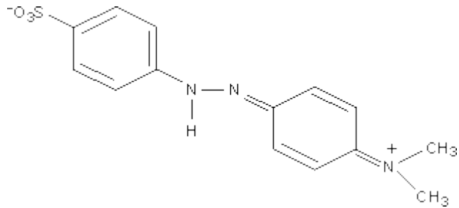
Gambar 6. Struktur metil orange
