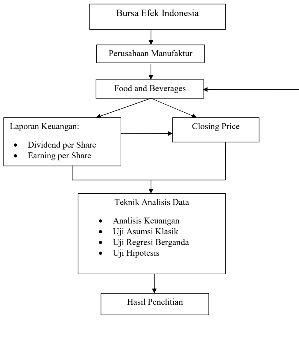
Gambar 2.1 Rerangka Pikir
