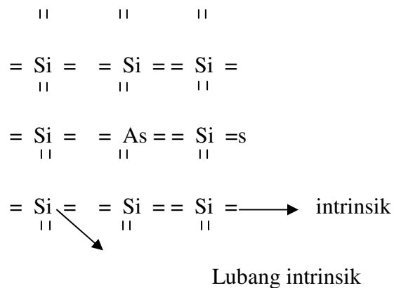
Gambar 4. Ikatan atom silikon dengan Arsenik bervalensi 5
