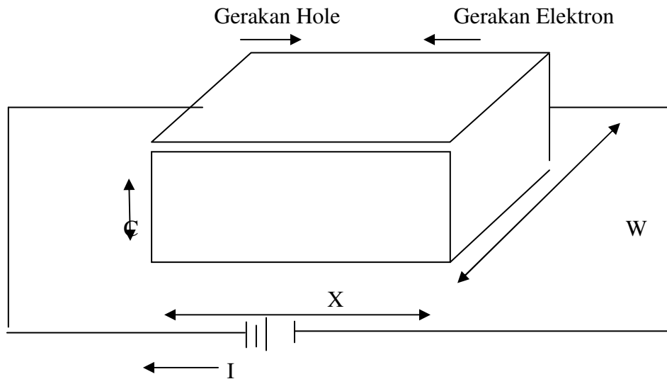
Gambar 14. Pergerakan hole dan elektron dalam sampel semikonduktor 27 .
