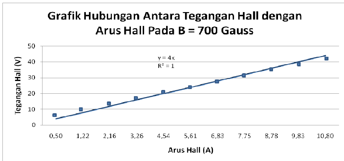
Gambar IV.2: Grafik Hubungan Antara Tegangan Hall ( V_H ) dengan Arus Hall ( I_H ).
