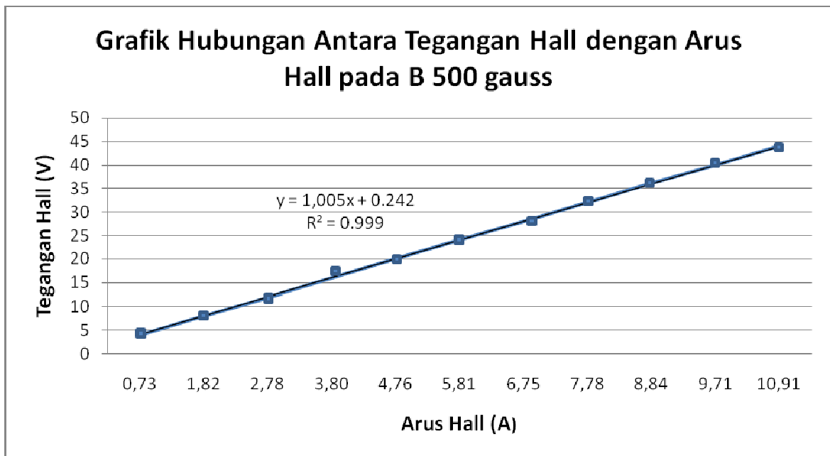
Gambar IV.1: Grafik Hubungan Antara Tegangan Hall (VH) dengan Arus Hall (IH).
