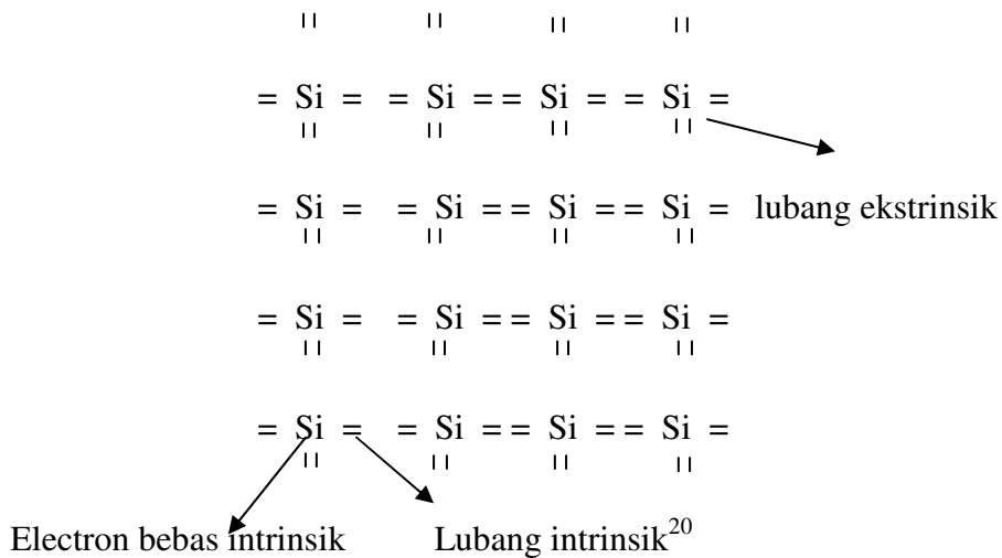
Gambar 5. Ikatan atom silikon dengan gallium bervalensi 3
