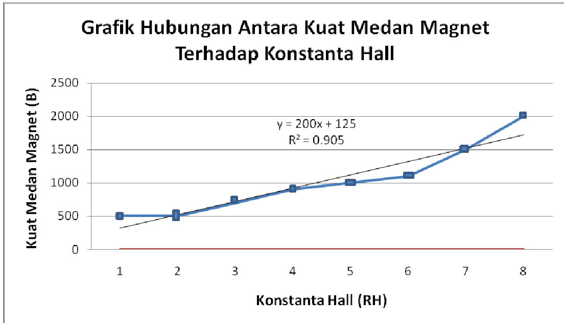
Gambar IV.3. Grafik Hubungan Antara Kuat Medan Magnet Terhadap Konstanta Hall
