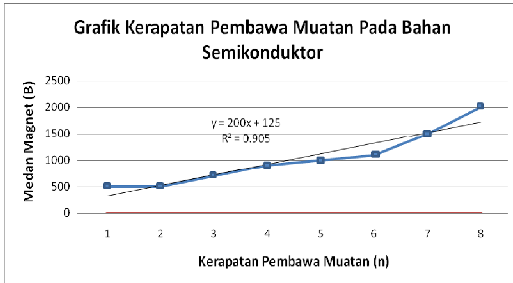
Gambar IV.3. Grafik hubungan medan magnet terhadap kerapatan pembawa muatan.
