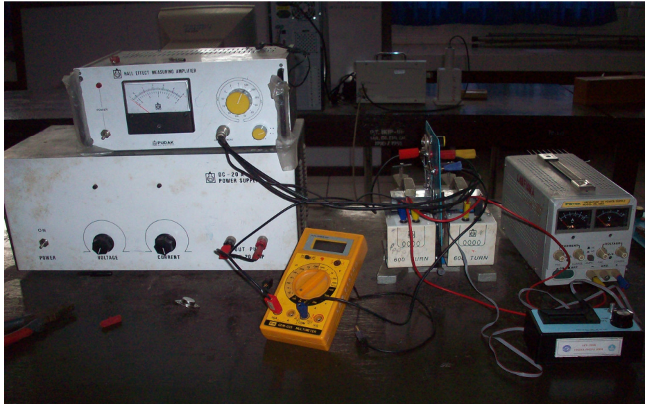
Gambar 16. Rangkaian Efek Hall
