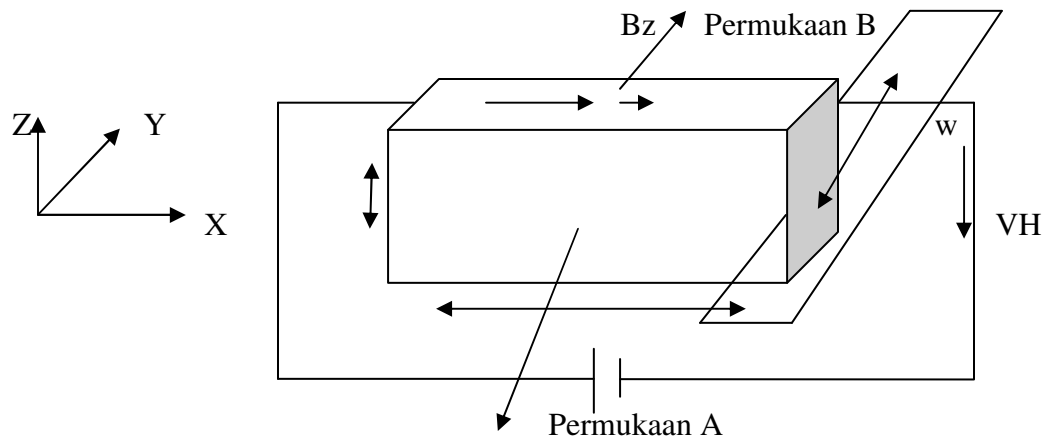
Gambar 11. Skema Efek Hall
