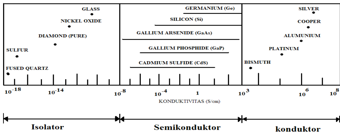
Gambar 15. Pembedaan material berdasarkan konduktivitas listrik 32
