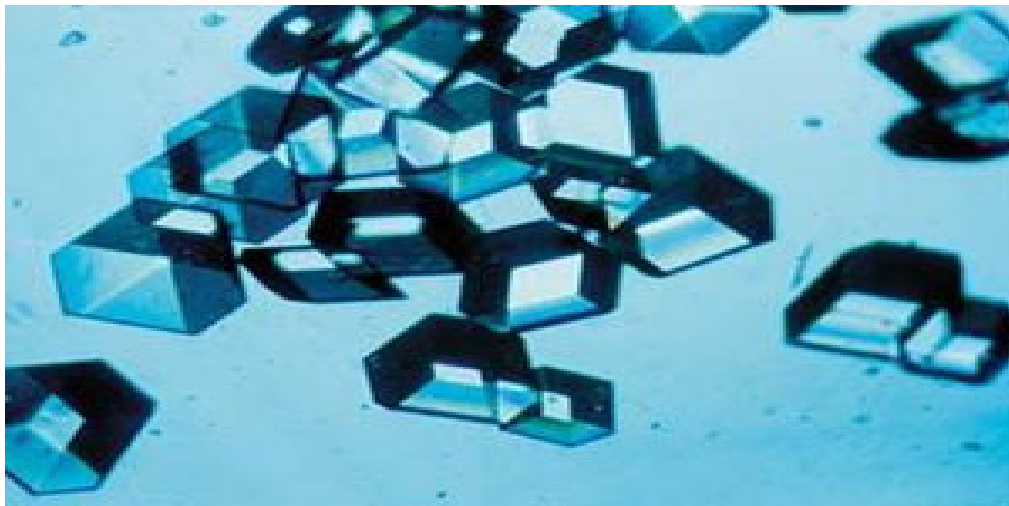
Gambar 7 Kristal insulin.
