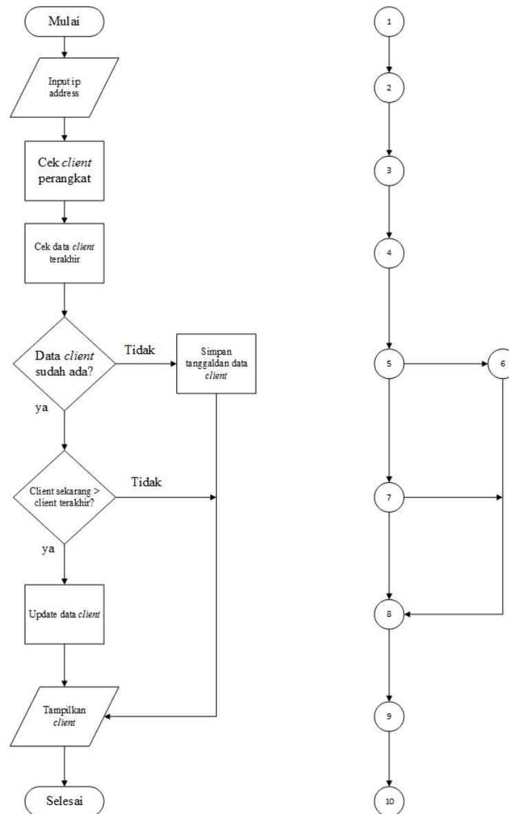
Gambar V.19 Pengujian Fungsi CheckClient
