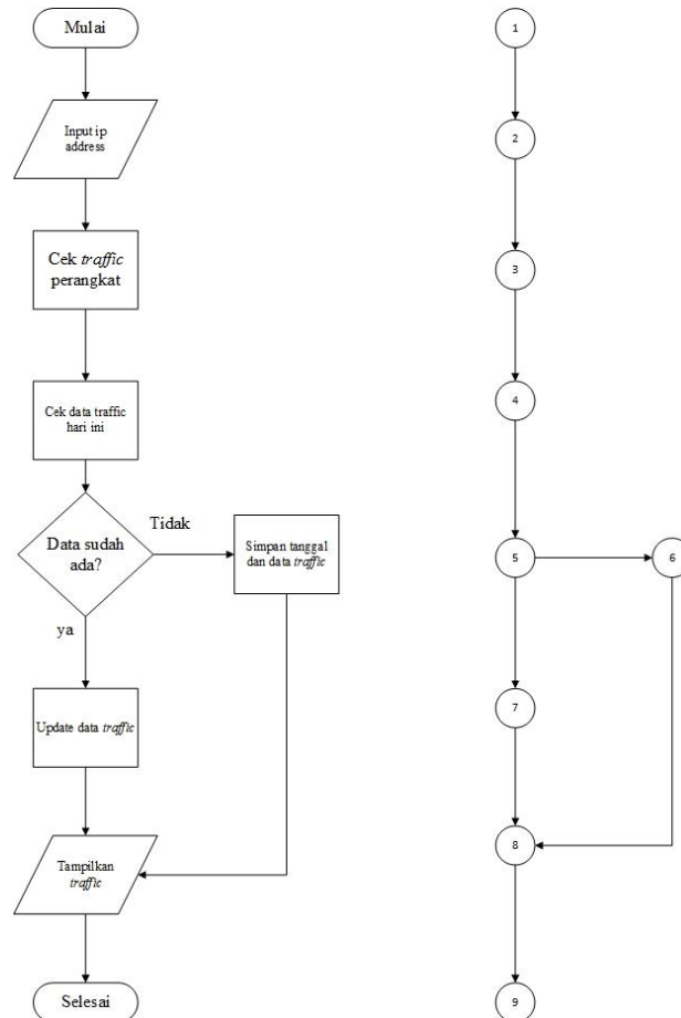
Gambar V.18 Pengujian Fungsi CheckTraffic
