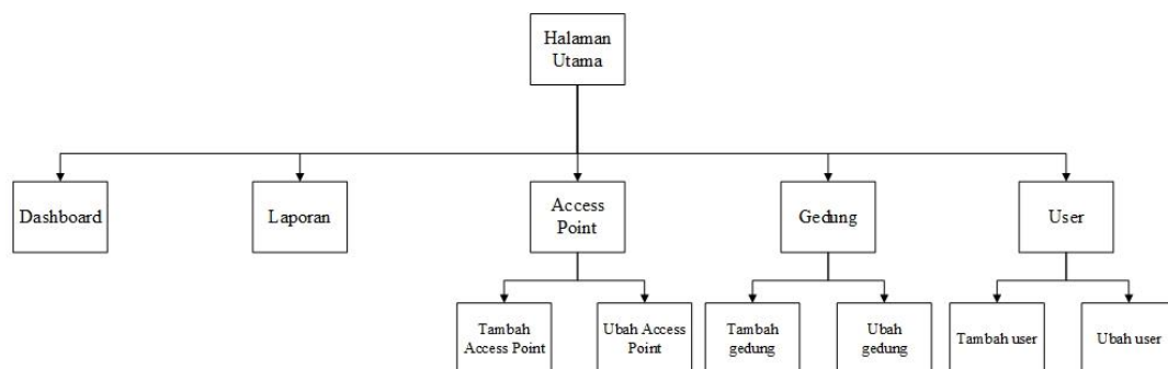
Gambar IV.8 Struktur Navigasi Halaman Panel Kontrol
