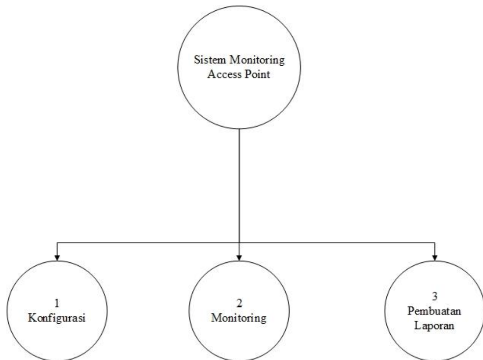
Gambar IV.4 Diagram Berjenjang
