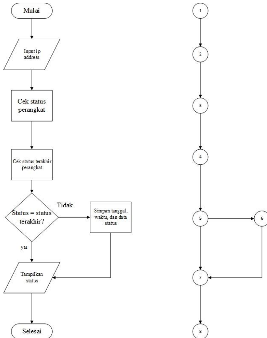
Gambar V.17 Pengujian Fungsi CheckStatus
