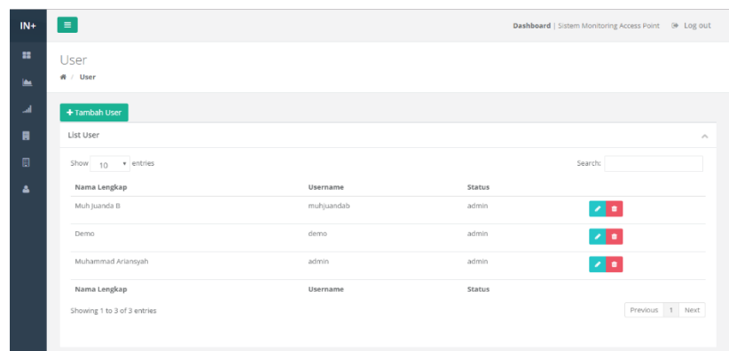
Gambar V.2 Antarmuka User
