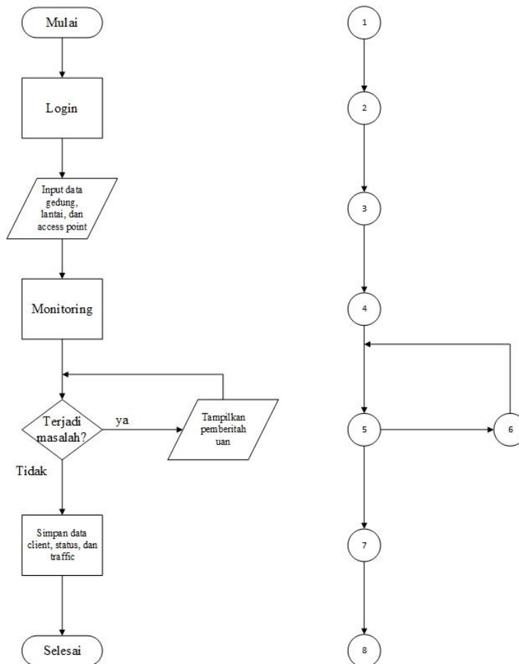
Gambar V.16 Pengujian Sistem
