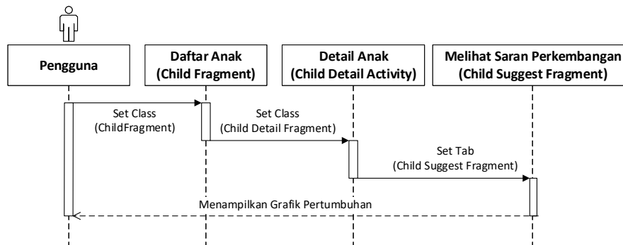
Gambar IV. 6 Sequence Diagram Melihat Saran Perkembangan
