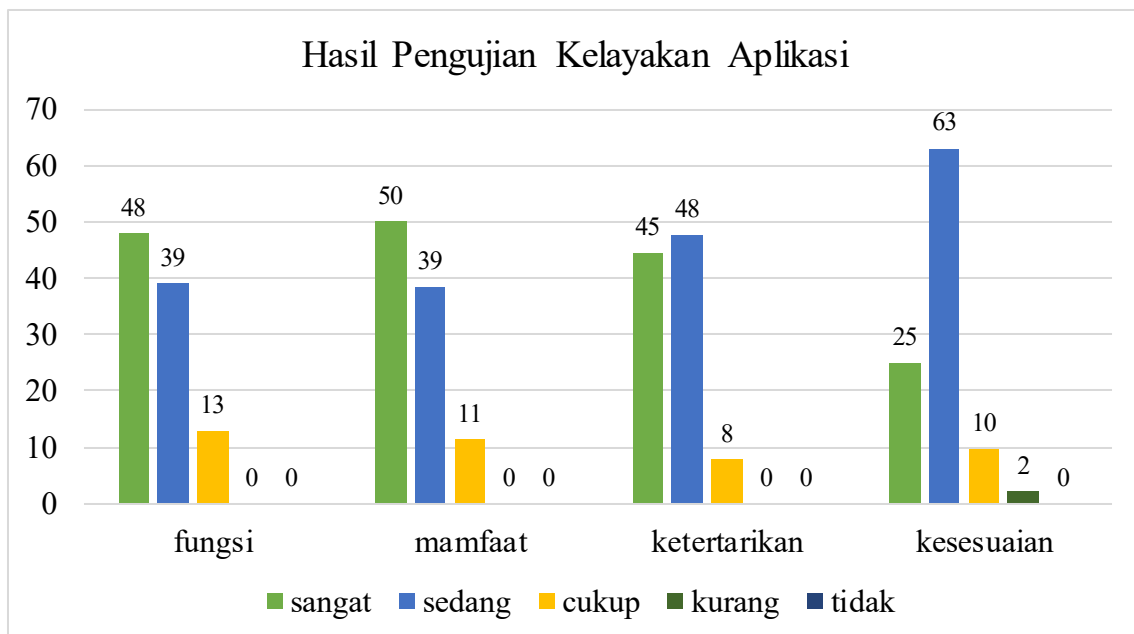
Gambar V. 15 Diagram Pengujian Kelayakan Aplikasi
