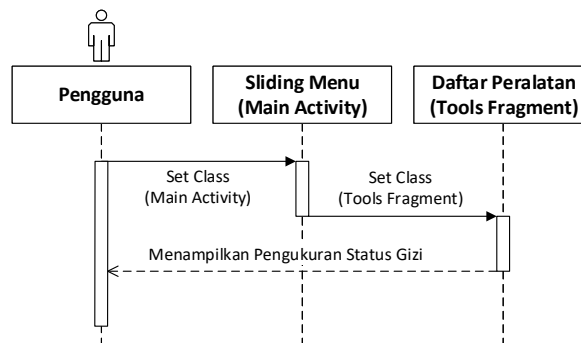
Gambar IV. 7 Sequence Diagram Melihat Daftar Peralatan
