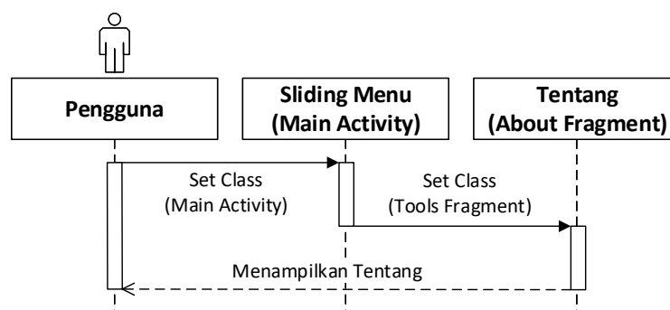
Gambar IV. 14 Sequence Diagram Membuka Tentang
