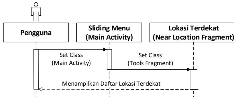
Gambar IV. 13 Sequence Diagram Membuka Lokasi Terdekat
