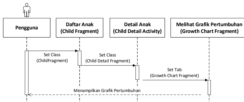
Gambar IV. 5 Sequence Diagram Melihat Grafik Perkembangan
