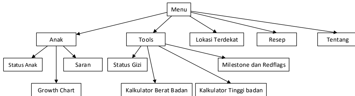
Gambar IV. 17 Struktur Navigasi
