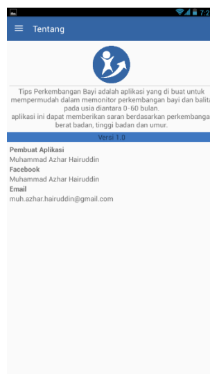
Gambar V. 9 Antarmuka Tentang
