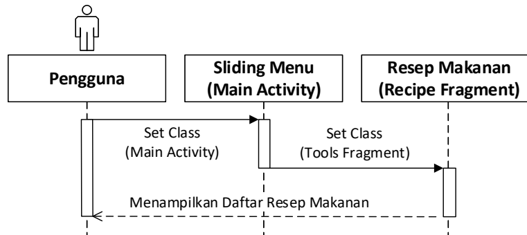
Gambar IV. 12 Sequence Diagram Membuka Resep Makanan
