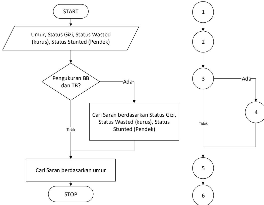
Gambar V. 13 Pengujian Pemberian Saran
