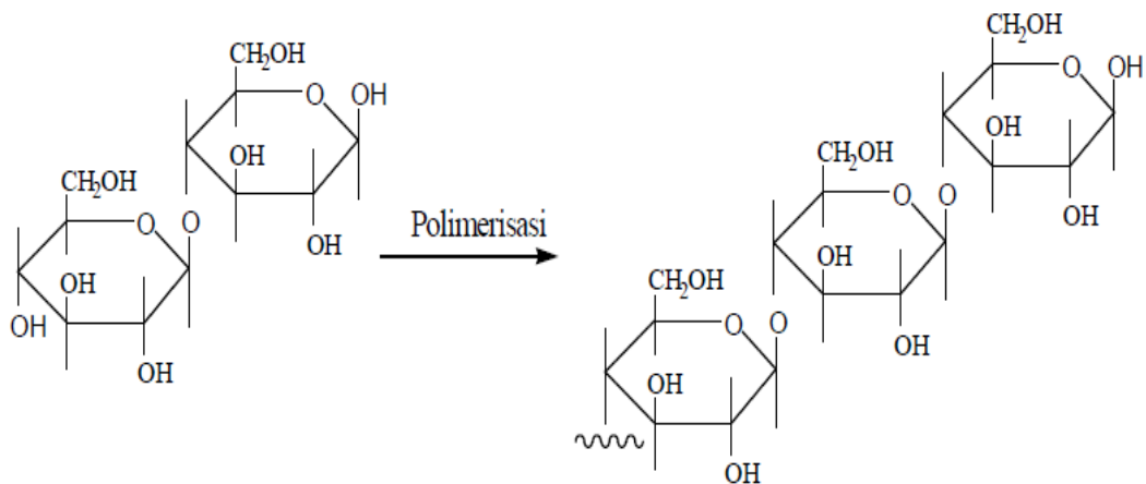
Gambar 6. Reaksi Polimerisasi terbentuknya selulosa
