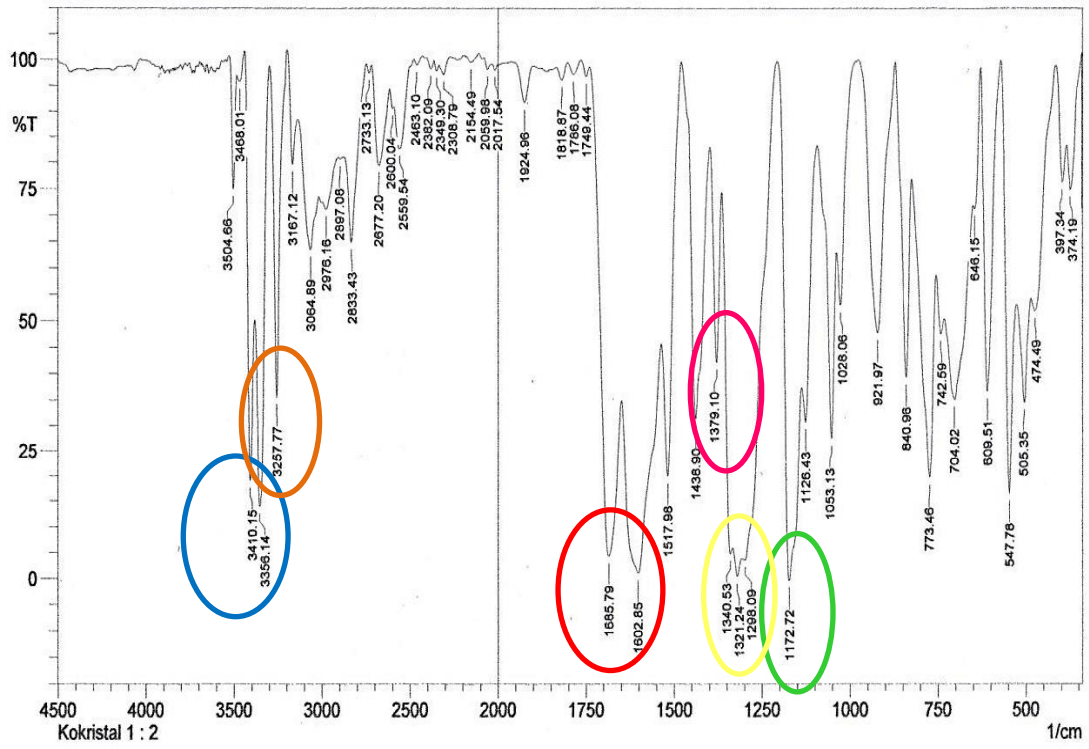
Gambar 22. Spektrum inframerah kokristal 1:2
