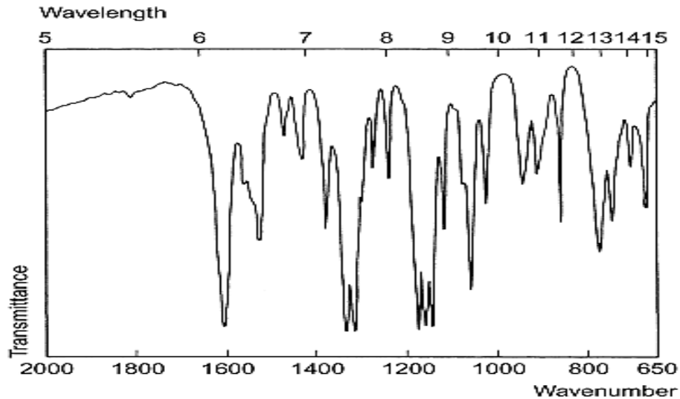
Gambar 3. Spektrum infra merah hidroklortiazid
