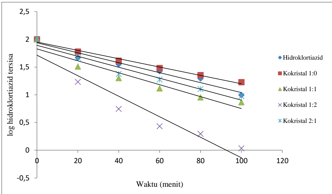
Gambar 26. Grafik plot orde satu
