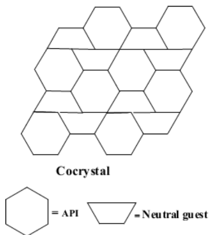
Gambar 8. Struktur kokristal
