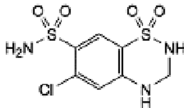
Gambar 1. Rumus struktur hidroklortiazid
