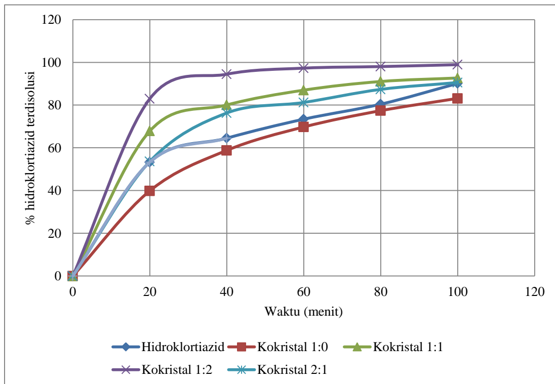
Gambar 16. Grafik profil disolusi hidrokloriazid dan kokristal
