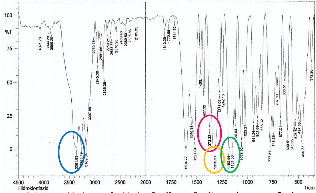
Gambar 20. Spektrum inframerah hidroklortiazid
