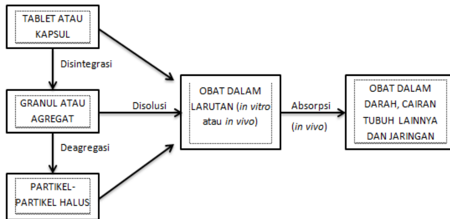
Gambar 12. Tahap-tahap disintegrasi, deagregasi, dan disolusi ketika obat meninggalkan suatu tablet atau matriks
