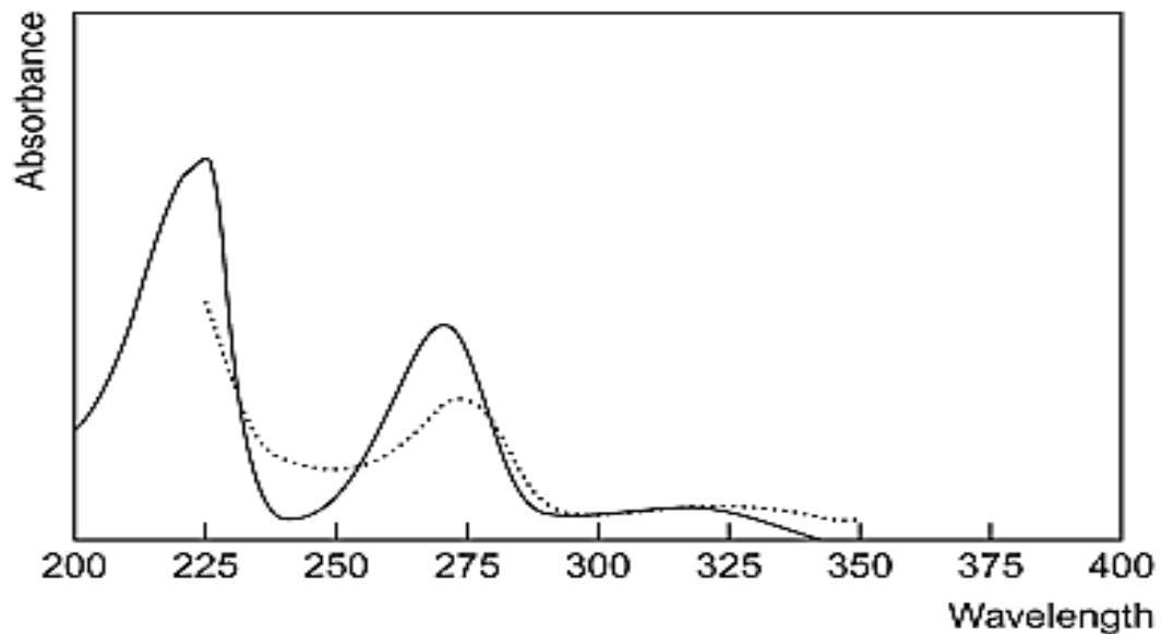
Gambar 2. Spektrum ultraviolet hidroklortiazid
