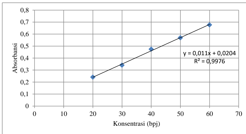
Gambar 15. Grafik kurva baku hidroklortiazid
