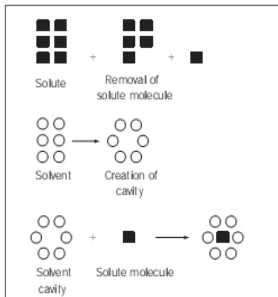
Gambar 11. Mekanisme pelarutan
