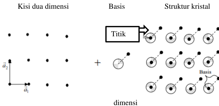
Gambar 7. Kisi dua
