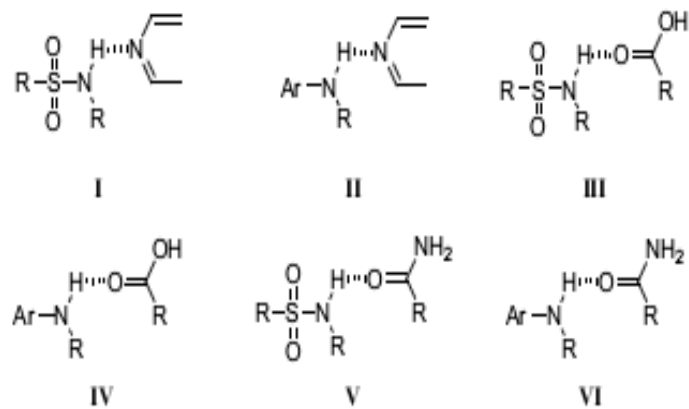
Gambar 10. Heterosinton supramolekuler yang mungkin untuk hidroklortiazid dengan koformernya.
