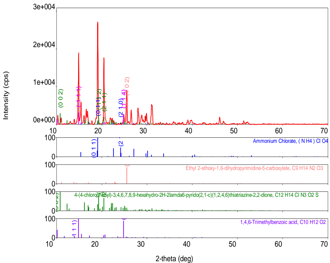
Lampiran 6. Hasil analisis kuantitatif XRD kokristal hidroklortiazid-asam para aminobenzoat 1:2
