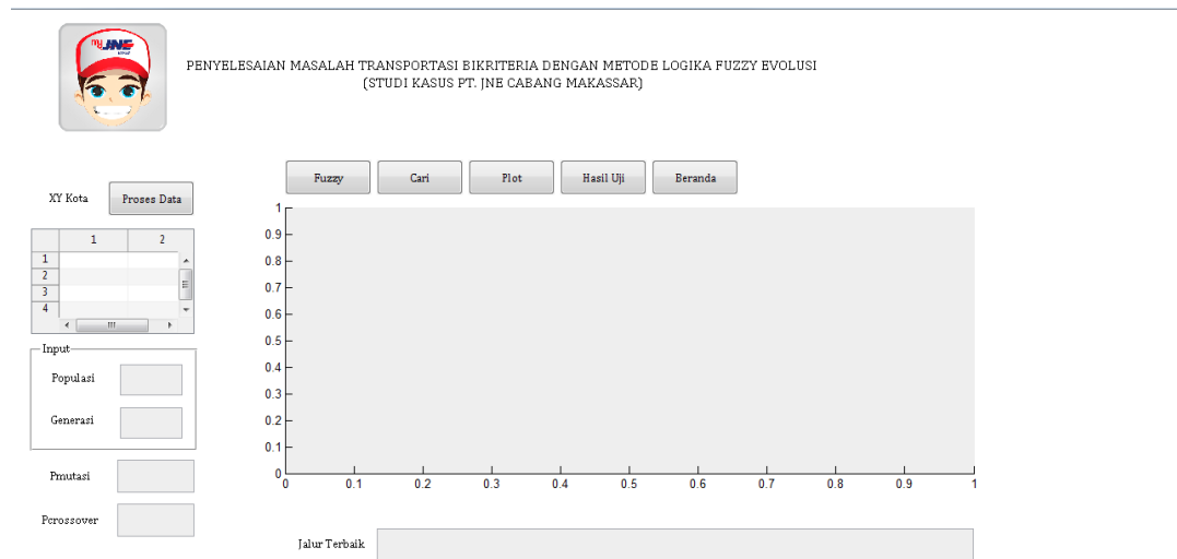
Gambar V.4 Antarmuka Sistem
