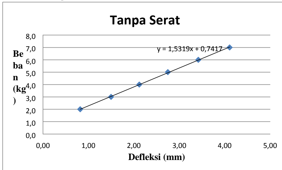
Grafik Hubungan antara Defleksi dan beban ( \Delta P/\Delta Y )
