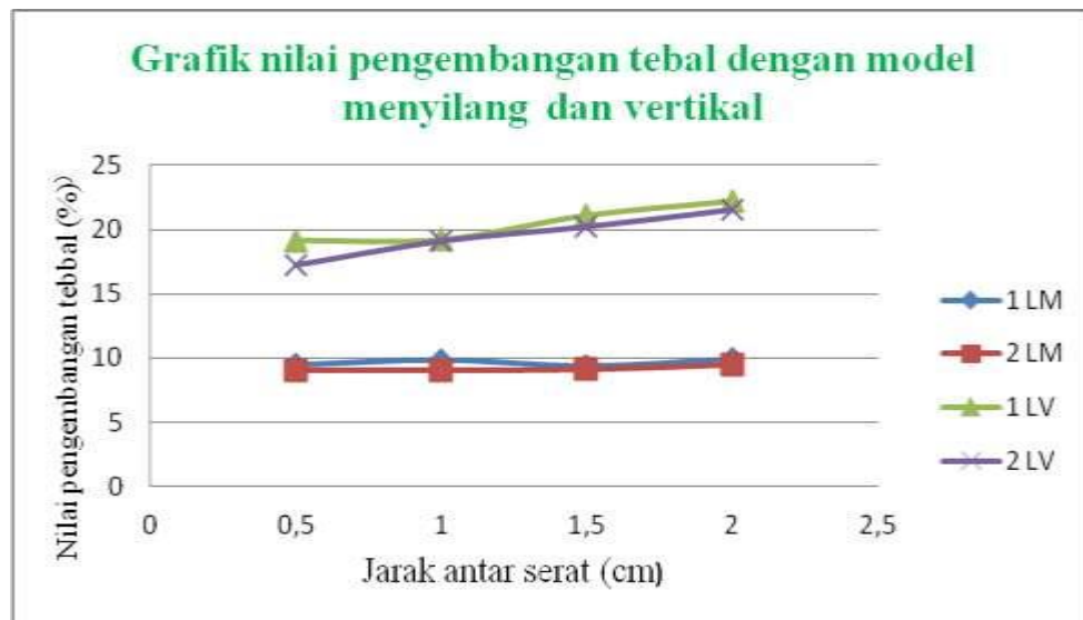
Gambar 4.2: Grafik nilai pengembangan tebal dengan model menyilang dan vertikal
