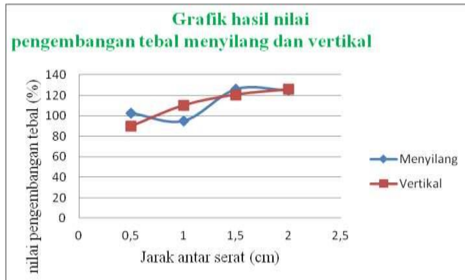
Gambar 4.3: Grafik hasil nilai pengembangan tebal dengan model menyilang dan vertikal
