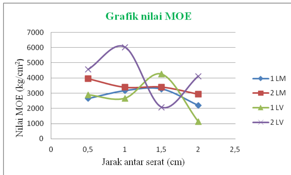
Gambar 4.4: Grafik nilai MOE dengan model menyilang dan vertikal
