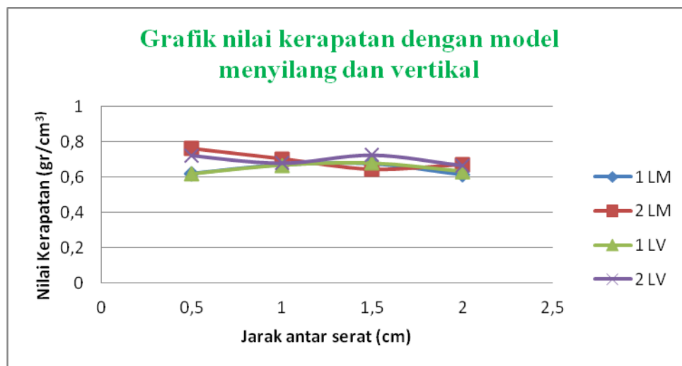
Gambar 4.1: Grafik nilai kerapatan dengan model menyilang dan vertikal
