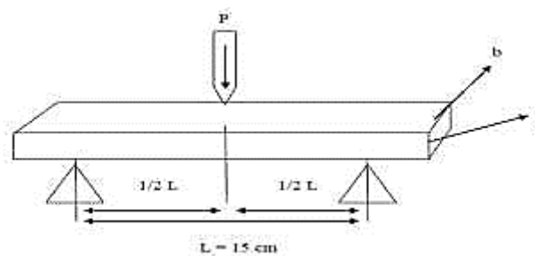
Gambar 3.4 : Pengujian MOE dan MOR
