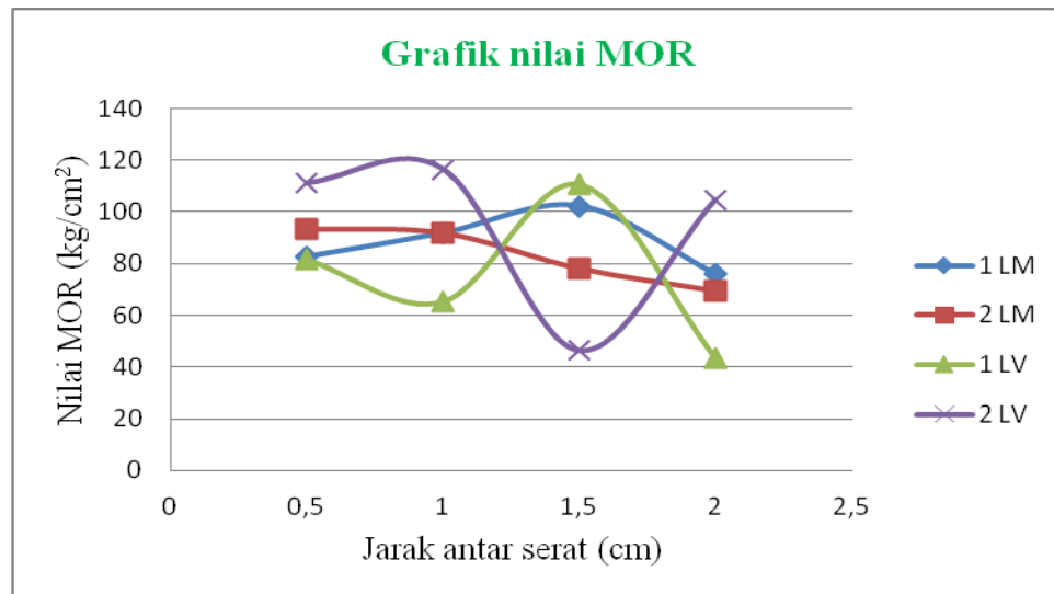
Gambar 4.5: Grafik uji MOR dengan model menyilang dan vertikal
