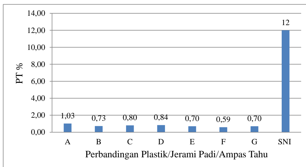
Grafik IV.3: Hasil pengujian pengembangan tebal
