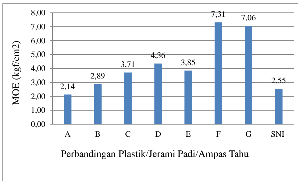
Grafik IV.4: Hasil pengujian modulus elastisitas (MOE)
