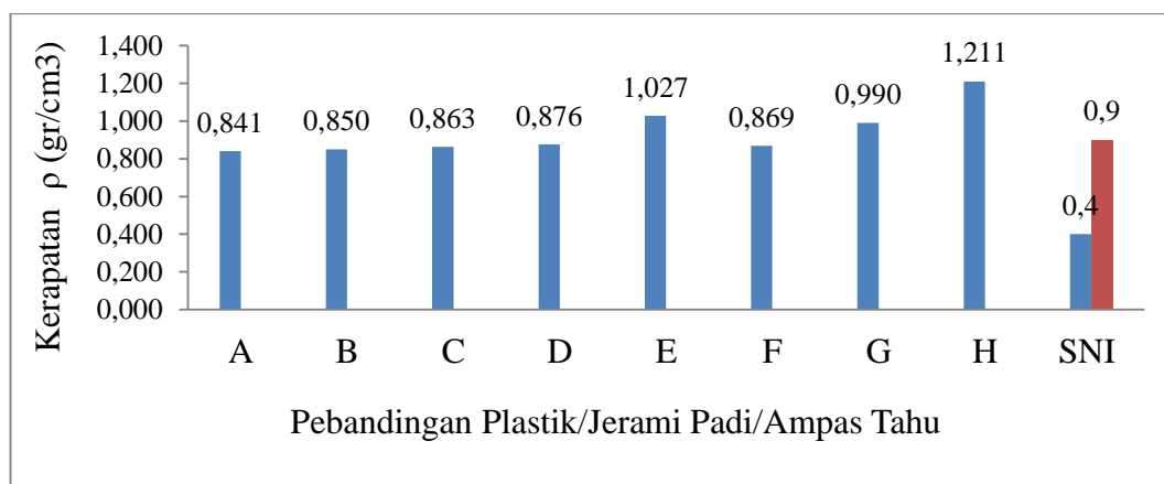
Grafik IV.1: Hasil pengujian kerapatan
