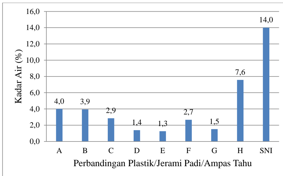
Grafik IV.2: Hasil pengujian kadar air
