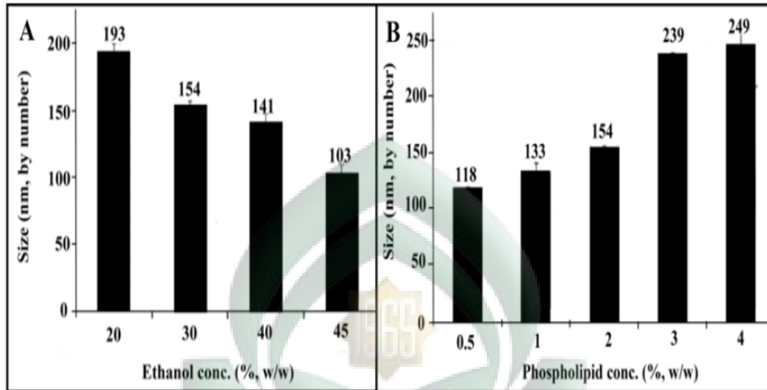
Gambar 6. Ukuran vesikel etosom mengandung 2% fosfatidilkolin kedelai, 30% etanol dan air diamati dengan DLS. (A) Pengaruh konsentrasi etanol pada ukuran vesikel. (B) Pengaruh konsentrasi fosfatidilkolin pada ukuran vesikel (Limsuwan, 2012)
