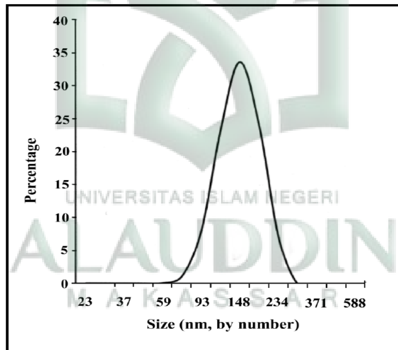
Gambar 5. Ukuran vesikel etosom terdiri dari 2% fosfatidilkolin kedelai, 30% etanol dan air yang diamati menggunakan DLS. (Limsuwan, 2012)
