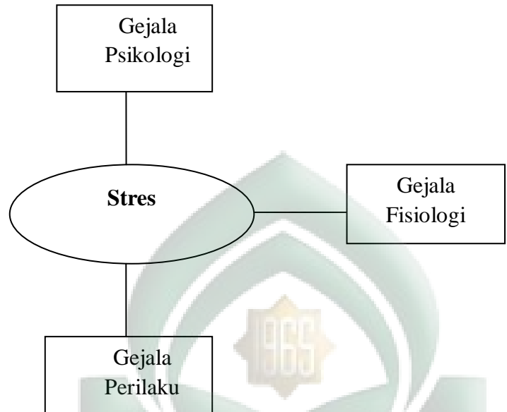
Gambar 1. Kerangka Teori
