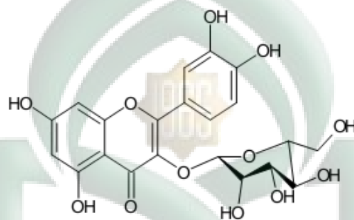
Gambar 4. Senyawa Morin
