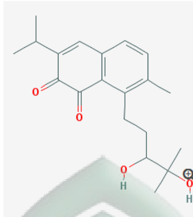
Gambar 9. Senyawa Salvicine
