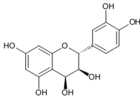
Gambar 7. Senyawa Leucocyanidin
