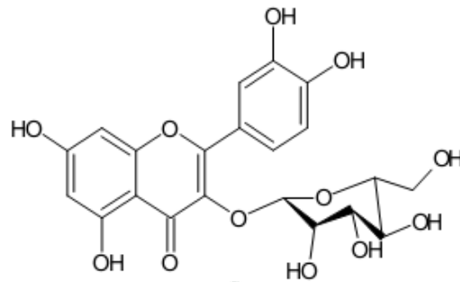
Gambar 3. Senyawa Isoquercetin
