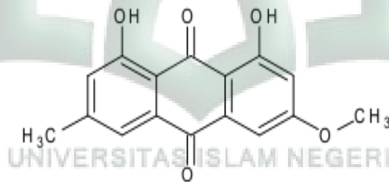
Gambar 5. Senyawa Physicion
