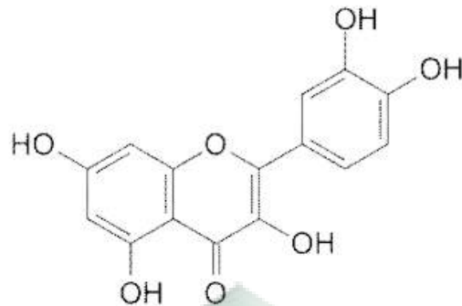
Gambar 2. Senyawa Quercetin
