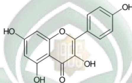
Gambar 8. Senyawa Kaempferol
