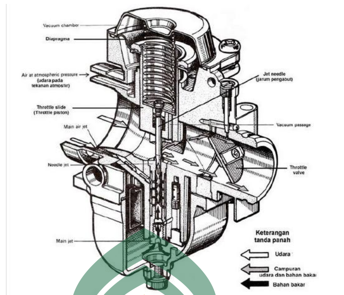
Gambar 2.3 Cara Kerja Karburator
