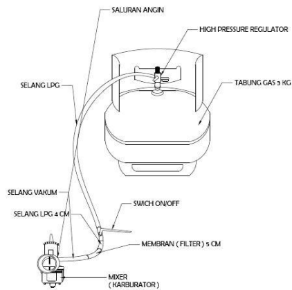
Gambar 4.1 Skema Rangkaian Konverter
