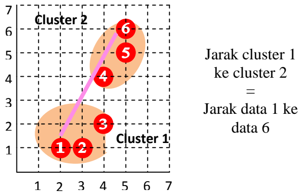
Gambar 1.4 Ilustrasi Complete Linkage
