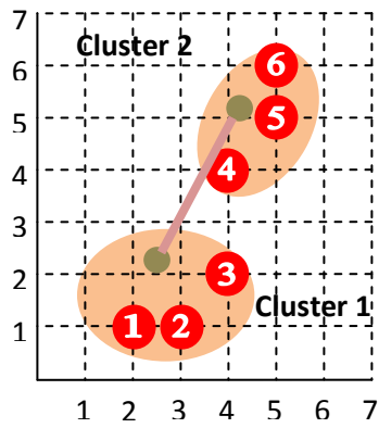
Gambar 1.6 Ilustrasi Centroid Linkage
