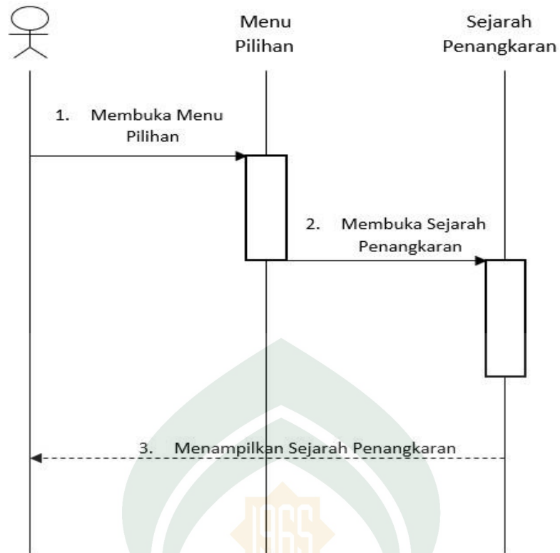
Gambar IV.9. Sequence Diagram untuk melihat menu Sejarah
