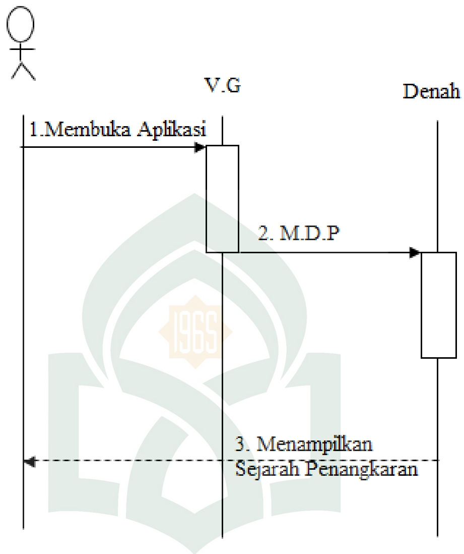
Gambar IV.6. Sequence Diagram untuk menjalankan Denah penangkaran satwa Bontomarannu Education Park
