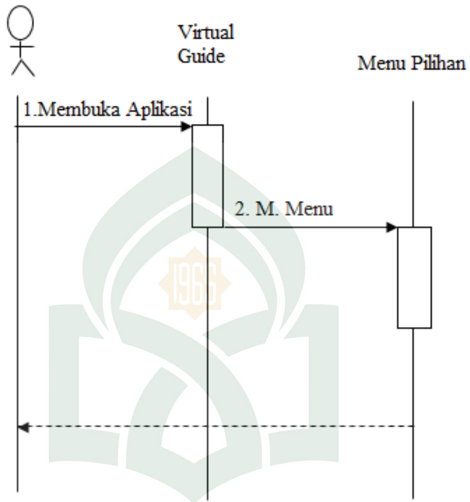
Gambar IV.7. Sequence Diagram untuk menjalan Menu Bontomarannu Education Park
