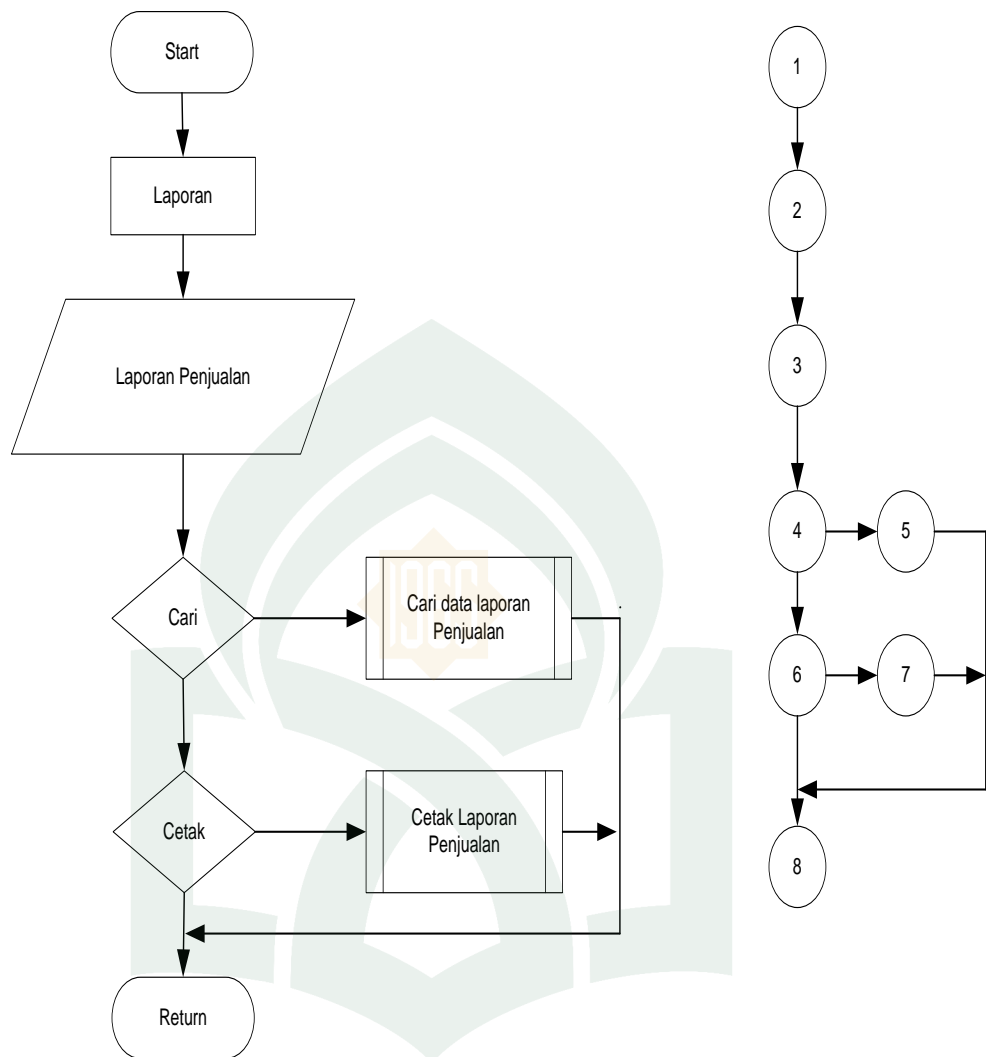
UNIVERSITAS ISLAM NEGERI Gambar V.29 Flowchart dan Flowgraph Sub Menu Laporan Penjualan
