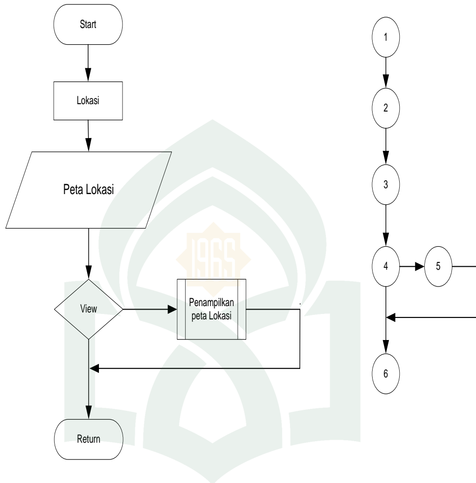
Gambar V.3 Flowchart dan Flowgraph Menu Lokasi
