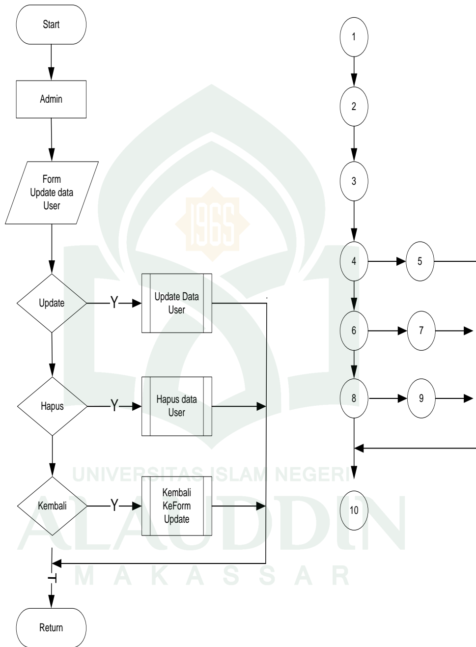
Gambar V.19 Flowchart dan Flowgraph Sub Menu User Aplikasi Form
