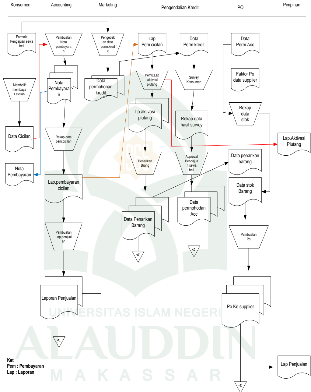
Gambar IV.1 Alur Sistem Yang Sedang Berjalan
