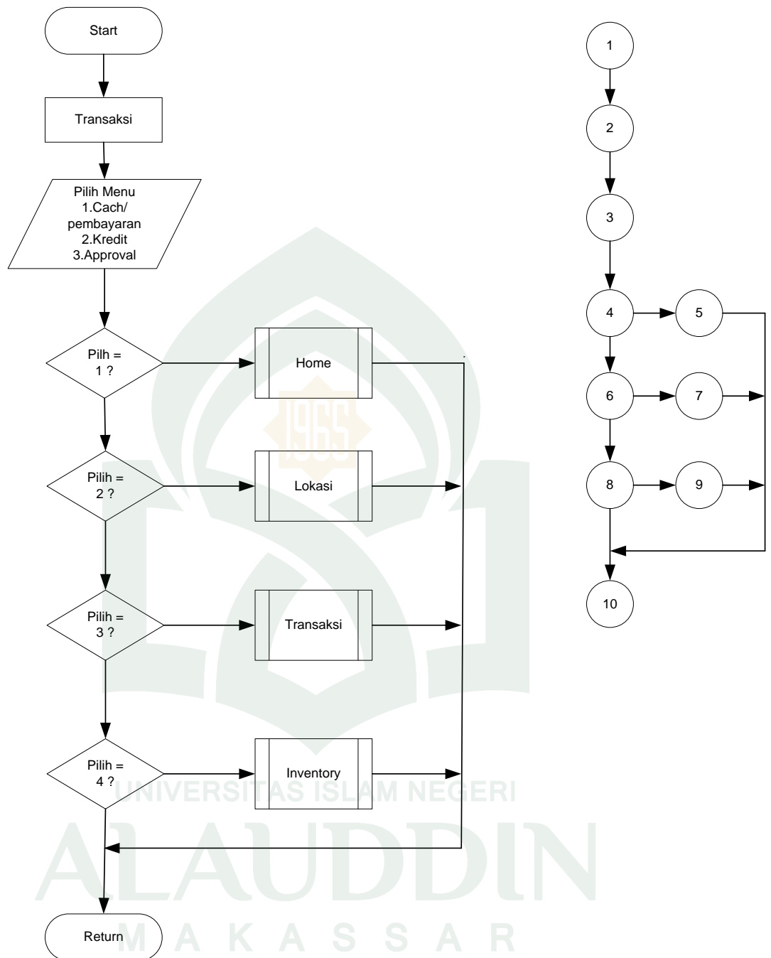
Gambar V.4 Flowchart dan Flowgraph Menu Transaksi
