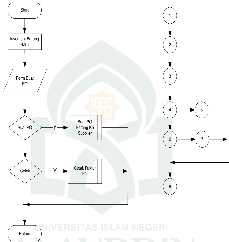
Gambar V.13 Flowchart dan Flowgraph Sub Menu Inventory Barang Baru Form Buat PO
