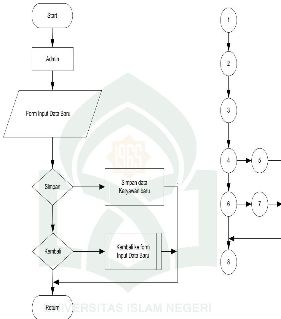
Gambar V.18 Flowchart dan Flowgraph Sub Menu User Aplikasi Form Input Data Baru
