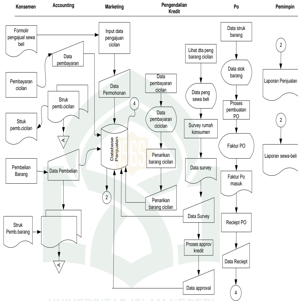
Gambar IV.2 Alur Sistem Yang Diusulkan
