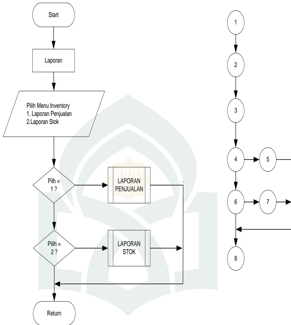
Gambar V.28 Flowchart dan Flowgraph Menu Laporan
