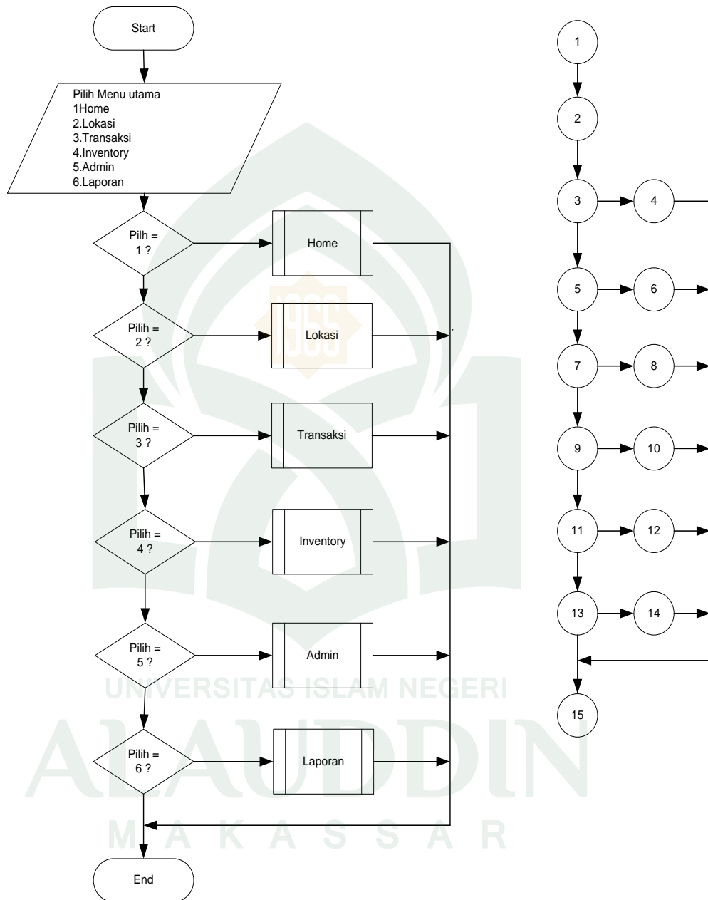
Gambar V.1 Flowchart dan Flowgraph Menu Utama
