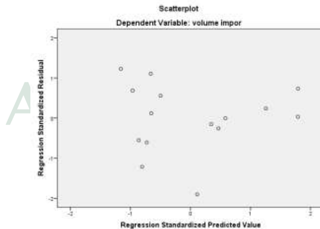
Gambar 5 Grafik Scatterplot
