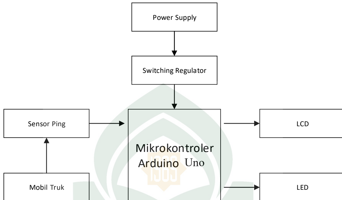
Gambar IV.1 Diagram Blok Sistem Alat
