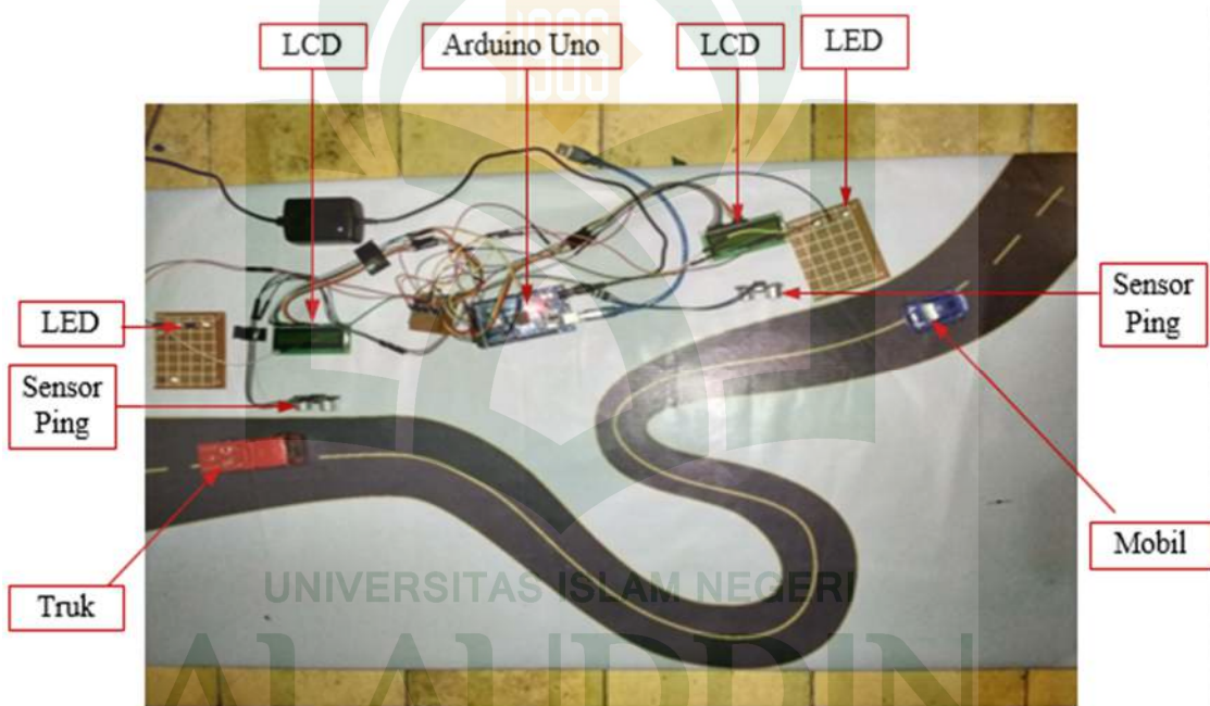
Gambar V.1 Hasil Rancangan Perangkat Keras Dari Sistem Pendeteksi Kemacetan pada jalur Maros Bone
