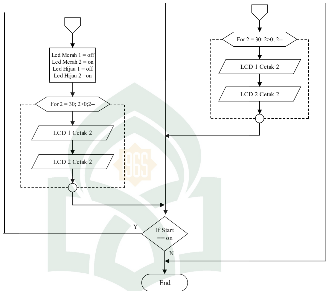
Gambar IV.8 Flowchart Sistem Pendeteksi Kemacetan Pada Jalur Poros Maros-Bone
