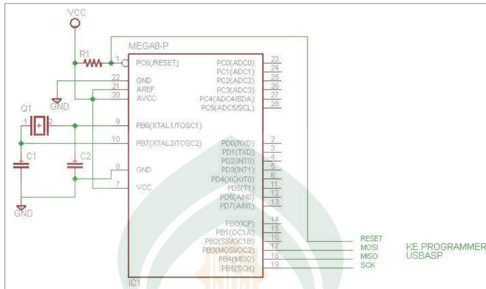
Gambar IV.5Rangkaian ArduinoUno
