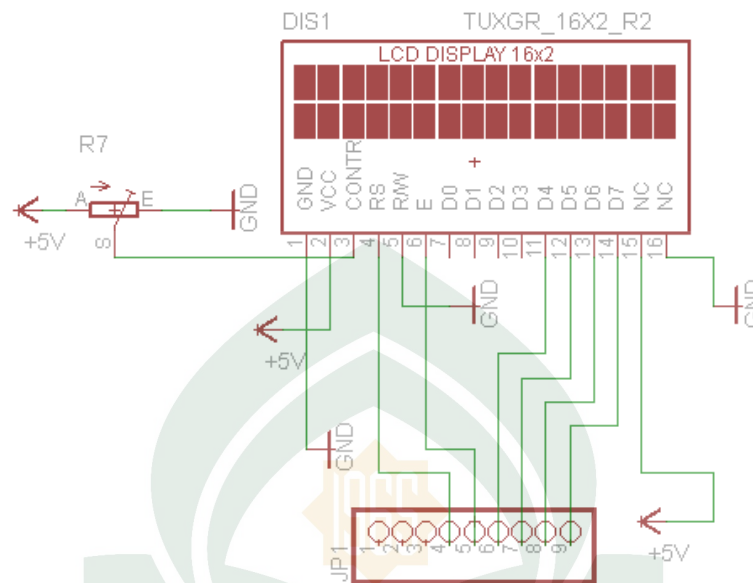
Gambar IV.6 Rangkaian LCD
