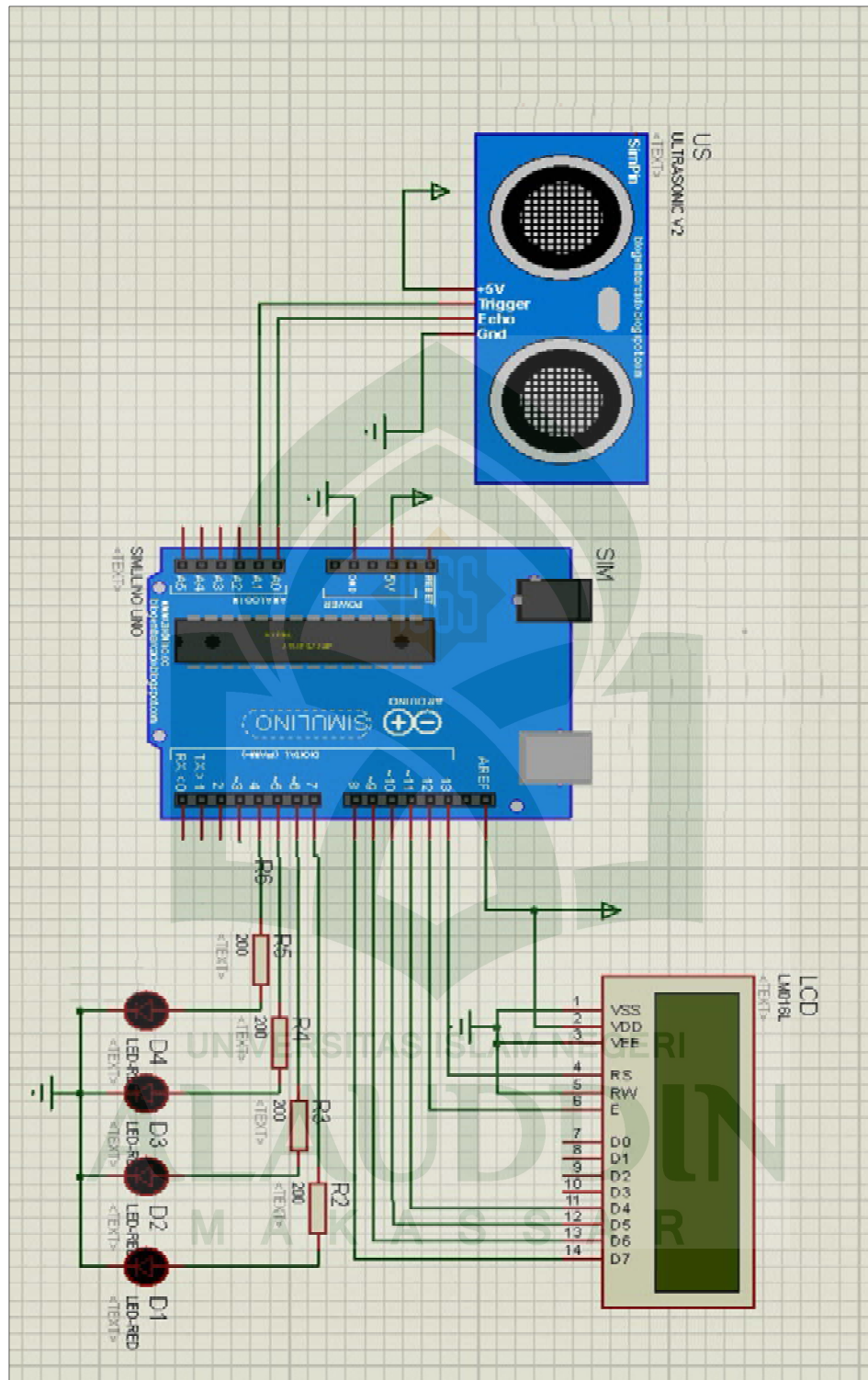
Gambar IV.7 Rangkaian Keseluruhan
