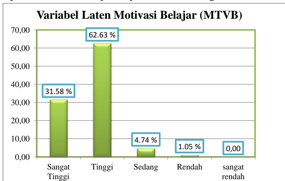
Gambar 4.3: Grafik Variabel laten Motivasi Motivasi Belajar (MTVB)
