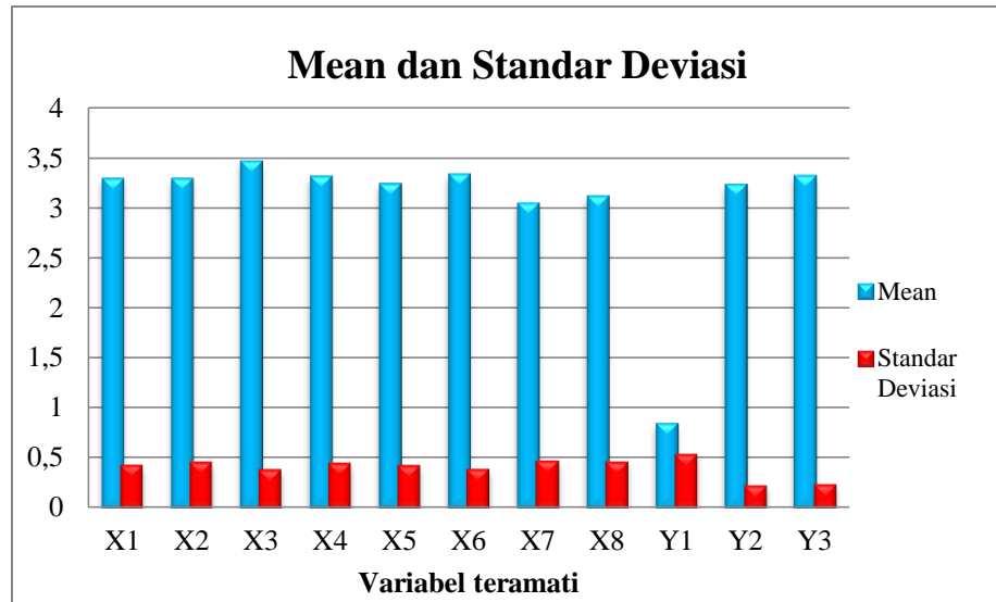
Gambar 4.1: Grafik Nilai Mean dan Standar Deviasi Variabel Teramati
