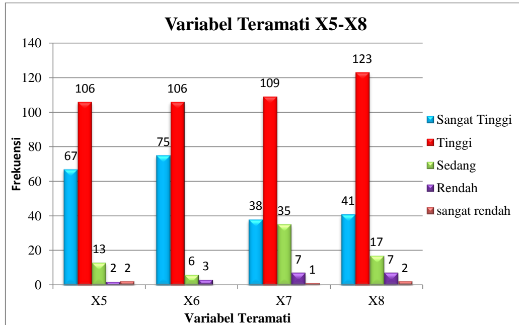
Gambar 4.3: Grafik Variabel Teramati X5-X8
