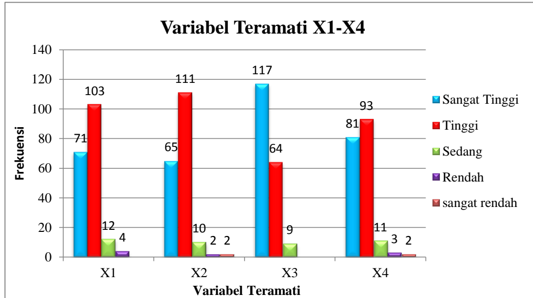
Gambar 4.2: Grafik Variabel teramati X1-X4
