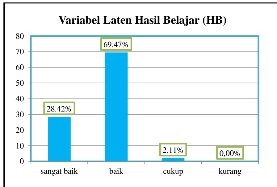
Gambar 4.5: Grafik variabel Laten Hasil Belajar (HB).
