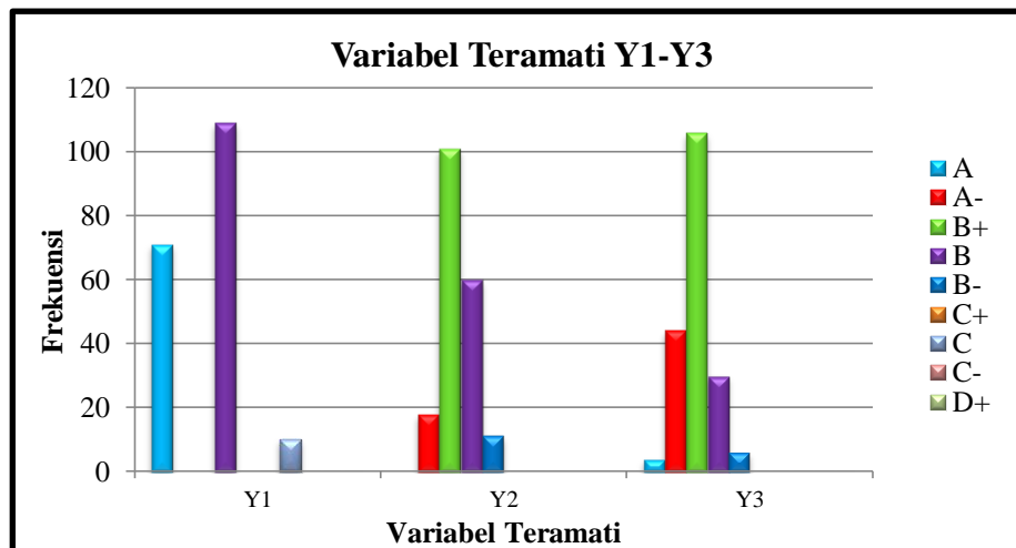
Gambar 4.4: Variabel Teramati Afektif ( Y_1 ), Kognitif( Y_2 ) dan Psikomotorik ( Y_3 )
