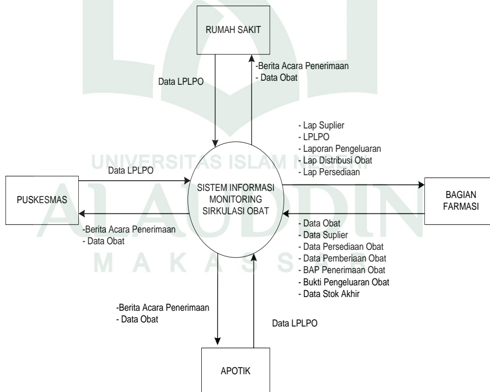
Gambar IV.3. Diagram Konteks
