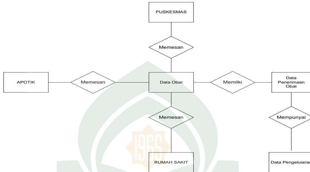
Gambar IV.8. ERD
