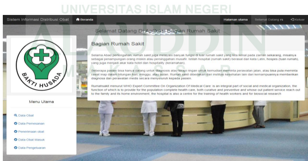
Gambar V.2 Menu Utama/Branda
