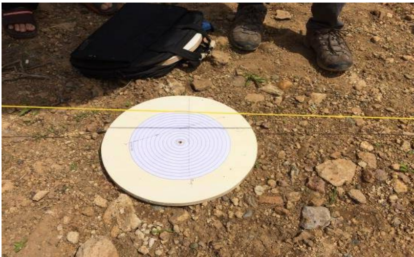
Gambar 2: Peletakan papan dan pemasangan tongkat
