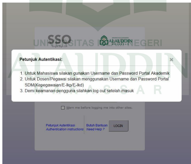
Gambar V.5 petunjuk autentikasi
