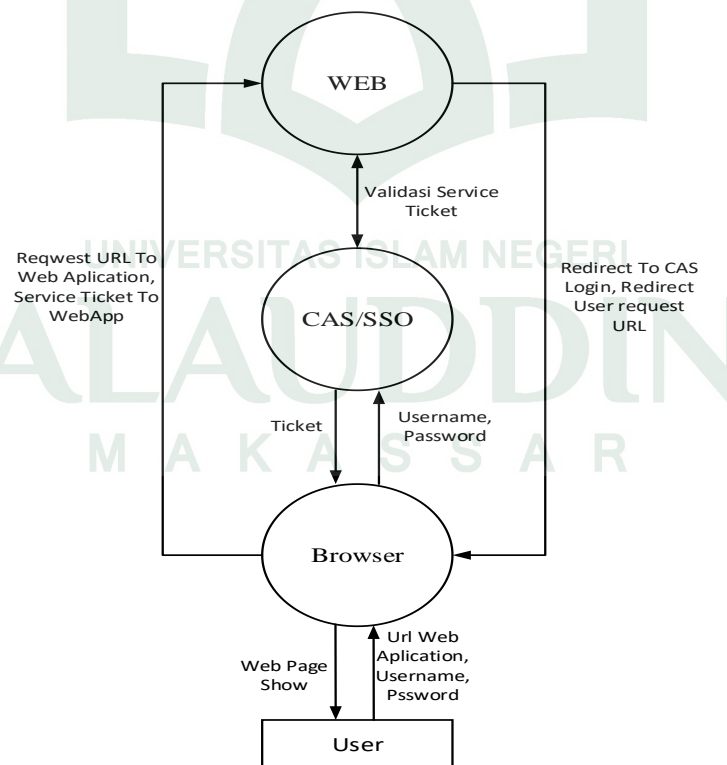
Gambar IV.3 Diagram Konteks
