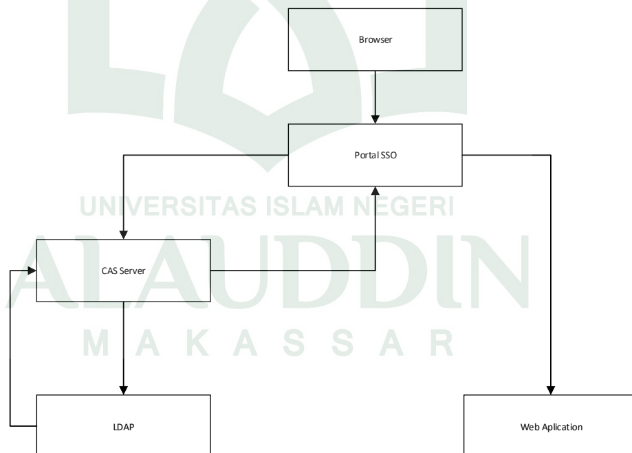
Gambar IV.7 Struktur Navigasi
