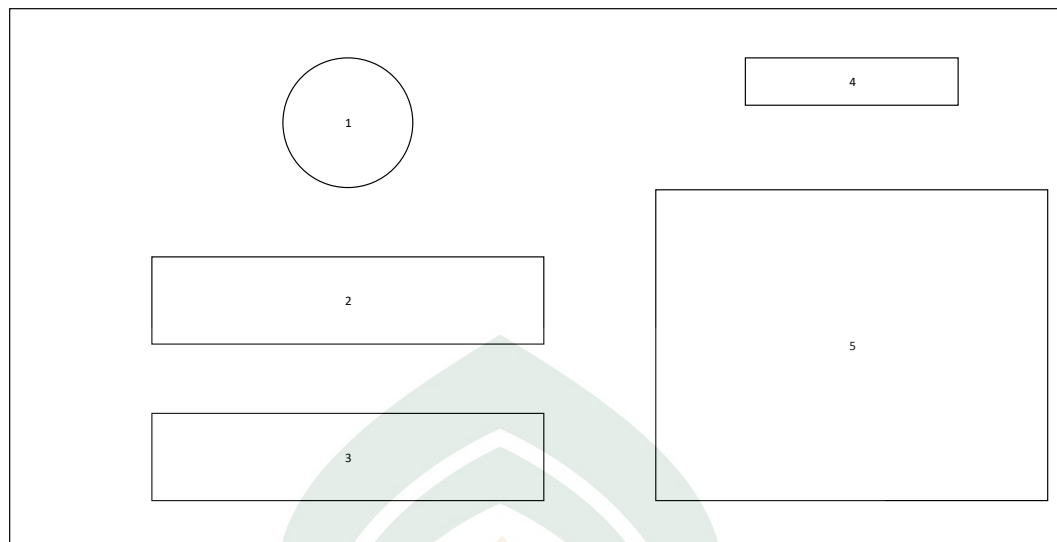
Gambar IV.8 Desain Antarmuka
