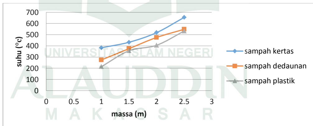
Grafik 4.3.3: Hubungan antara massa sampah terhadap suhu pembakaran.
