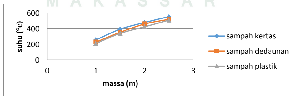
Grafik 4.3.4: Hubungan antara massa sampah terhadap suhu pembakaran.
