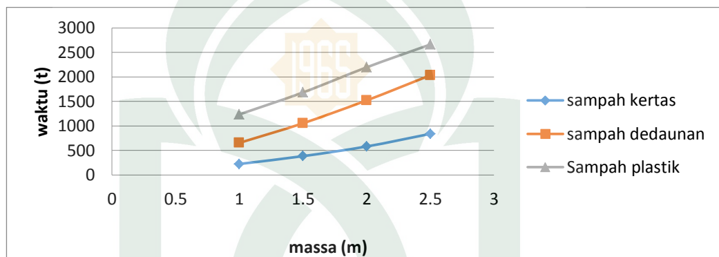
Grafik 4.3.1: Hubungan antara massa sampah terhadap lamanya waktu pembakaran
