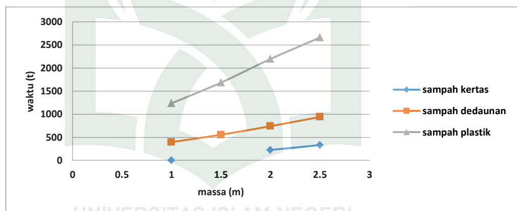
Grafik 4.3.2 : Hubungan antara massa sampah terhadap lamanya waktu pembakaran
