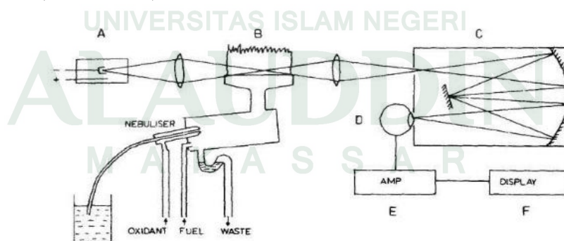
Gambar 2.8 skema spektrofotometer serapan atom
