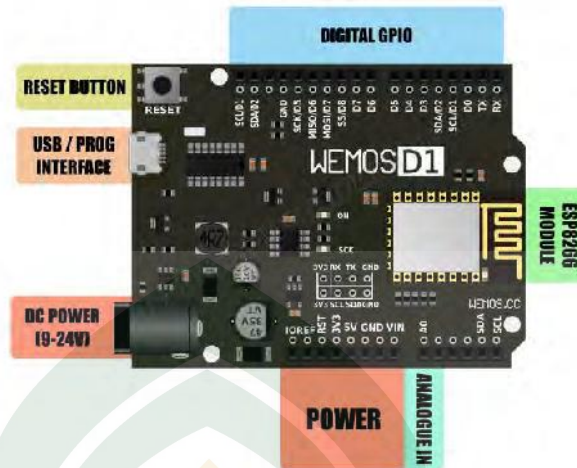
Gambar II.4 Skema Mikrokontroler Wemos D1 Mini ( http://hobbycomponents.com/images/forum/wemos/Wemos_D1_HCWEMO0001_Diagram.png )
