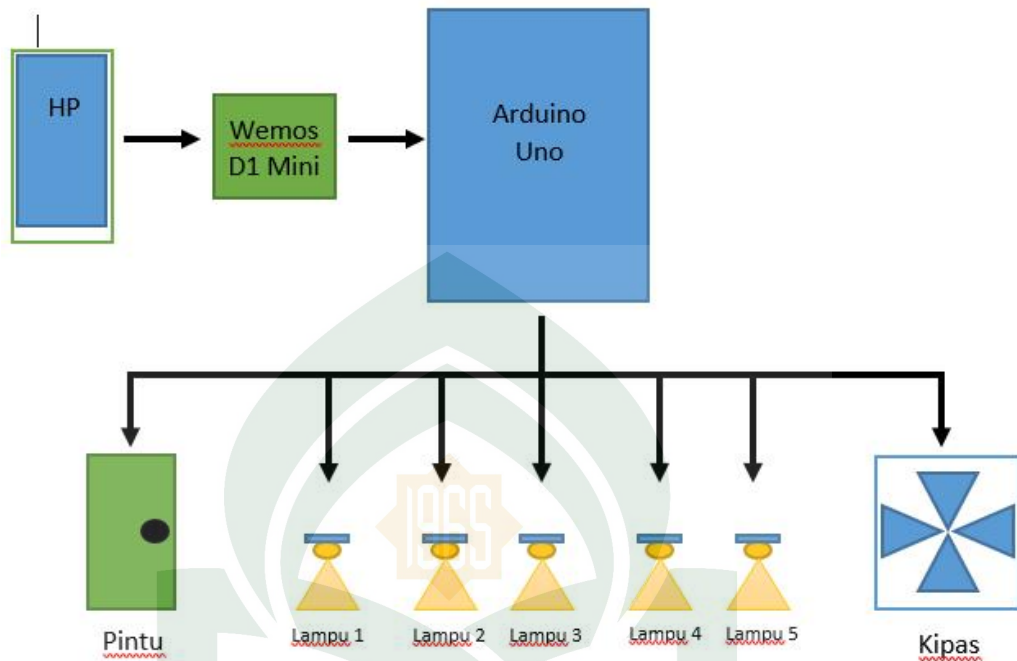
Gambar IV.6. Rancangan Mekanik Elektronika
