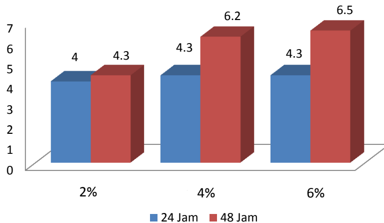
Gambar 4.4 Diameter Zona Hambat Ekstrak N-heksan Metode Evaporator Putar Vakum
