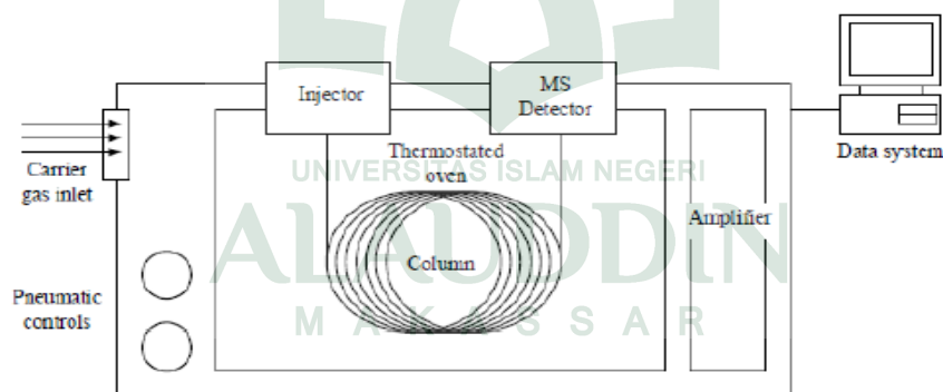
Gambar 2.5. Skema KGSM
