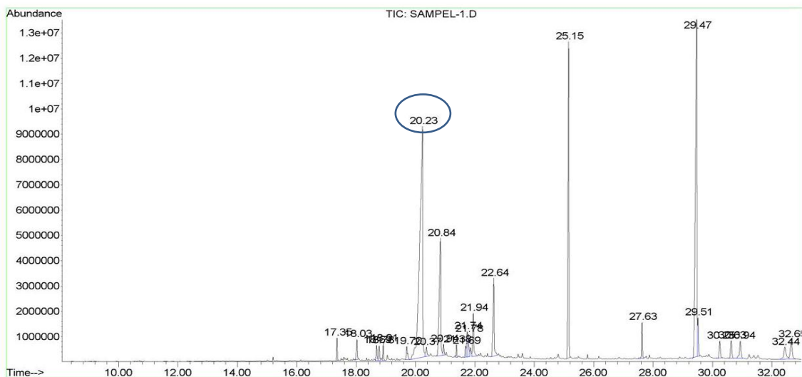
Gambar 4.6. Kromatogram KGSM Ekstrak Etil Asetat Alga Merah
