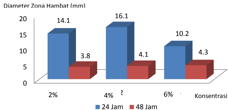
Gambar 4.2 Diameter Zona Hambat Ekstrak Etil Asetat Metode Evaporator Putar Vakum
