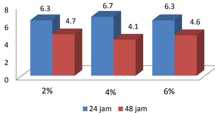
Gambar 4.3 Diameter Zona Hambat Ekstrak Metanol Metode Evaporator Putar Vakum
