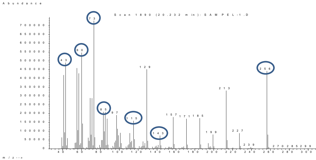
Gambar 4.7. Spektrum Massa Asam Heksadekanoat pada Waktu Retensi 20,23
