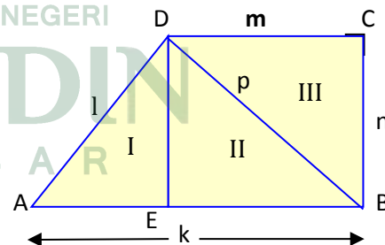
Gambar 7. Segiempat ABCD
