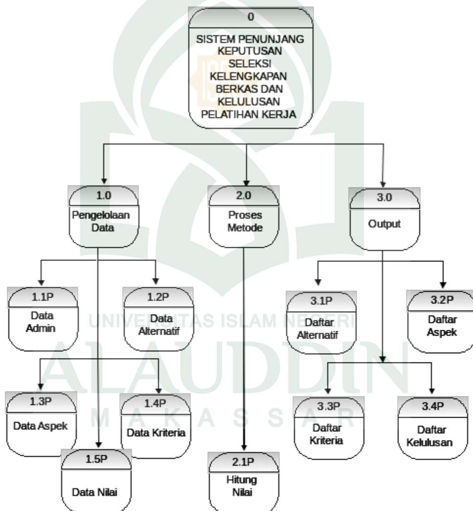
Gambar IV.7 Hirarki Input Proses Output
