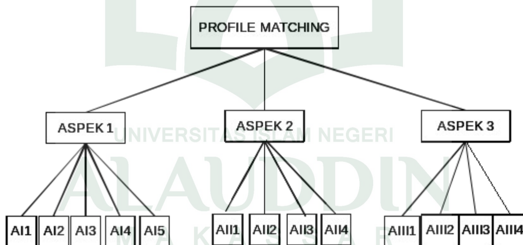
Gambar IV.3 Struktur Profile Matching
