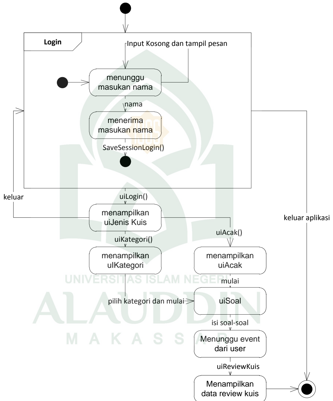
Gambar IV.3 Statechart Diagram Aplikasi Kuis Budaya Tradisional di Indonesia
