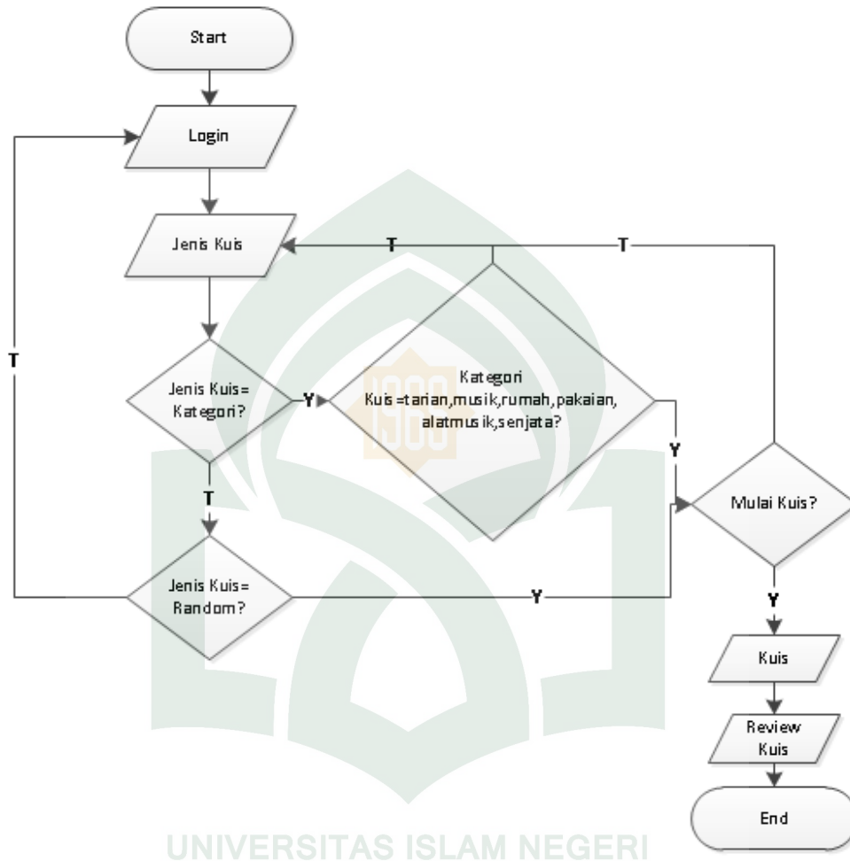
Gambar IV.4 Flowchart Aplikasi Kuis Budaya Tradisional di Indonesia
