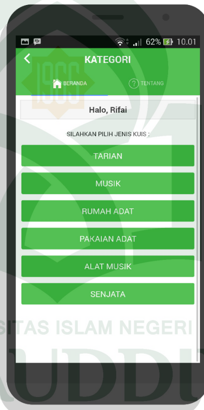
Gambar V.5 Antarmuka Kategori
