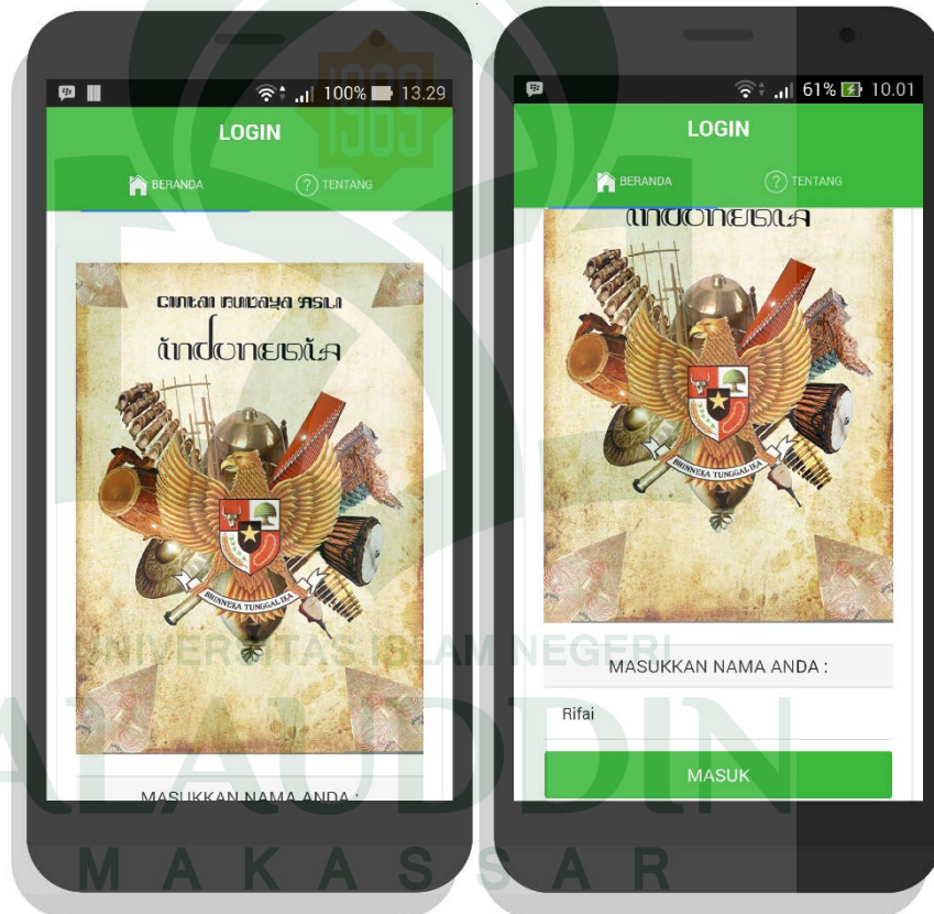
Gambar V.2 Antarmuka Login
