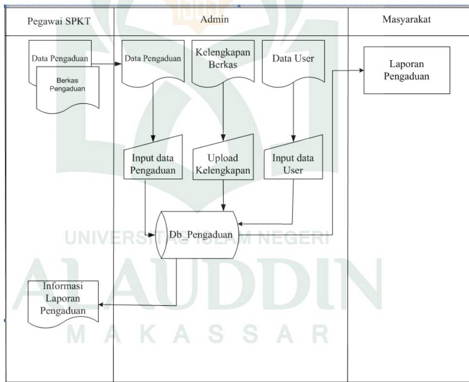
Gambar IV. 2 Flowmap Sistem yang sedang Diusulkan
