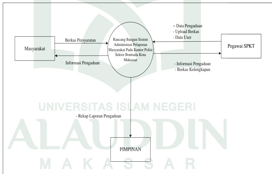
Gambar IV. 3 Diagram Konteks
