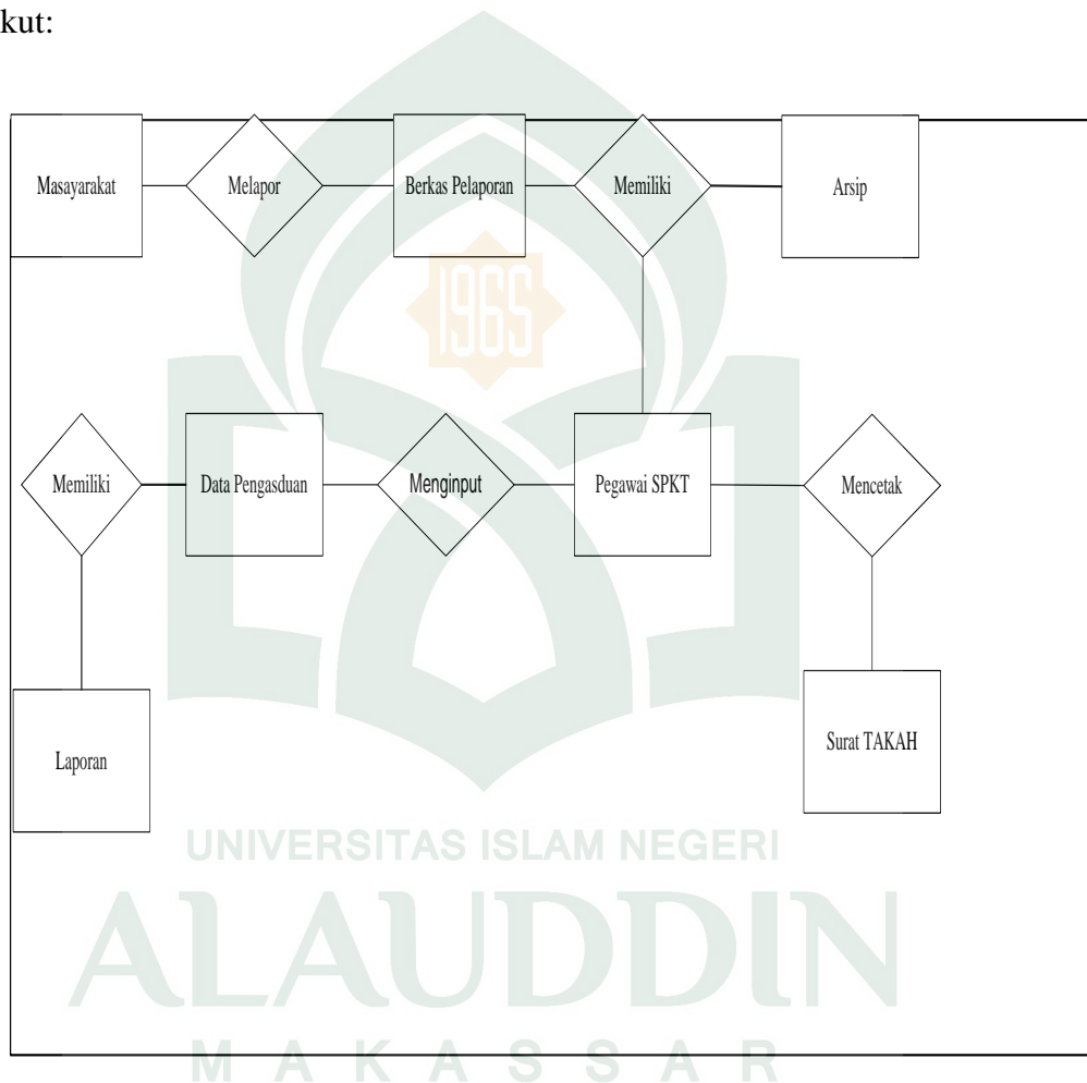
Gambar IV. 9 ERD
